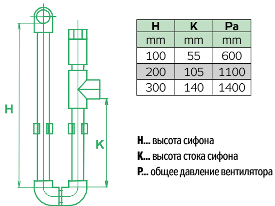
РИСУНОК 14 - ОТВОД КОНДЕНСАТА
