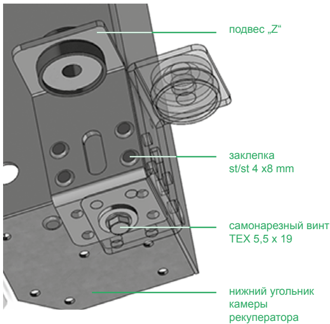
РИСУНОК 12 - МОНТАЖ НА ПОДВЕС Z
