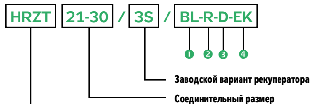
РИСУНОК 7 - ТИПОВОЕ ОБОЗНАЧЕНИЕ КАМЕРЫ РЕКУПЕРАТОРА
