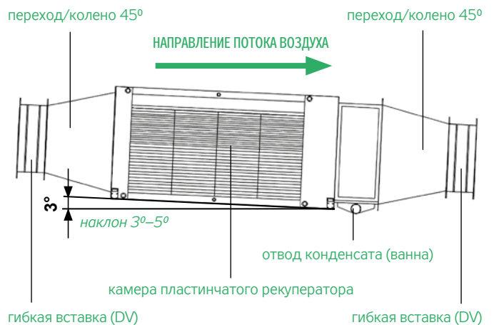
РИСУНОК 3 - ПОДВЕСКА КАМЕРЫ С ПОЛОЖИТЕЛЬНЫМ НАКЛОНОМ
