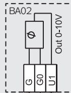
Připojení motoru a frekvenčního měniče rotačního výměníku
