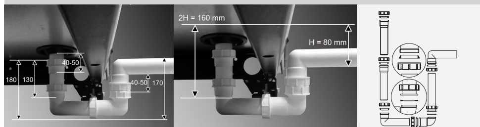
Obrázek 12 – Odvod kondenzátu
