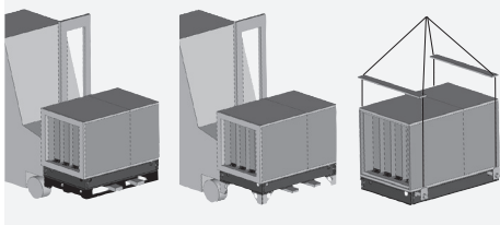
Obrázek 2 – strojní manipulace
