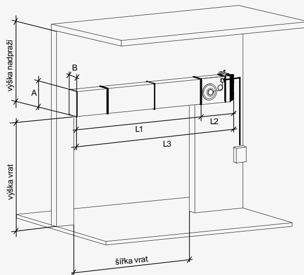
Horní – nad vratovým otvorem
