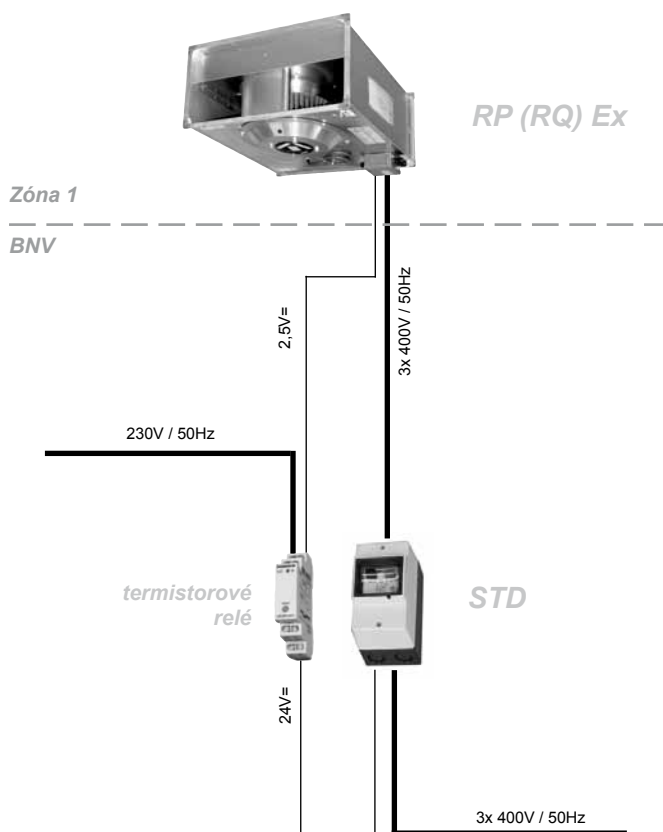
Obrázek 17 – zapojení ventilátoru
