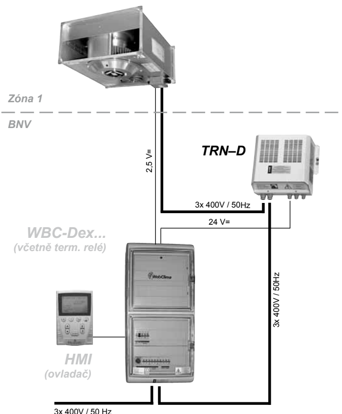
Obrázek 20 – zapojení ventilátoru
