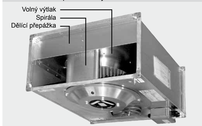
Obrázek 9 – uspořádání výtlačku ventilátoru
