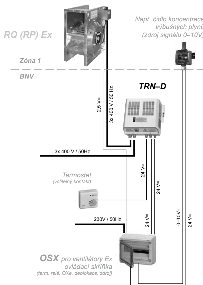
Obrázek 21 – zapojení ventilátoru
