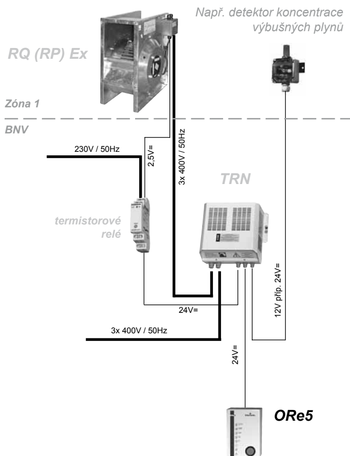
Obrázek 18 – zapojení ventilátoru
