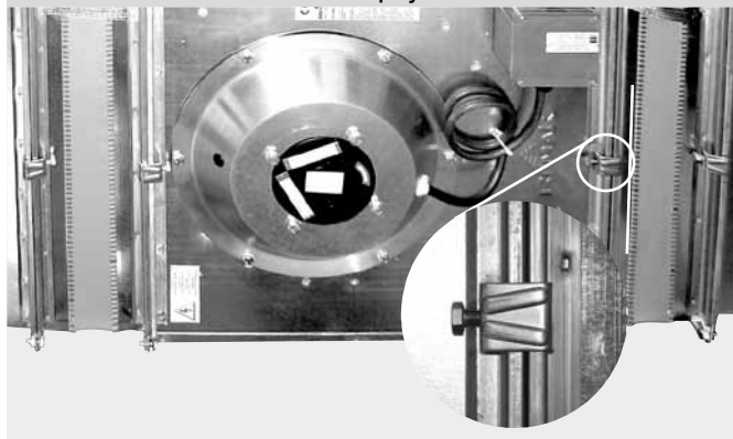
Obrázek 13 – šroubovací spoje
