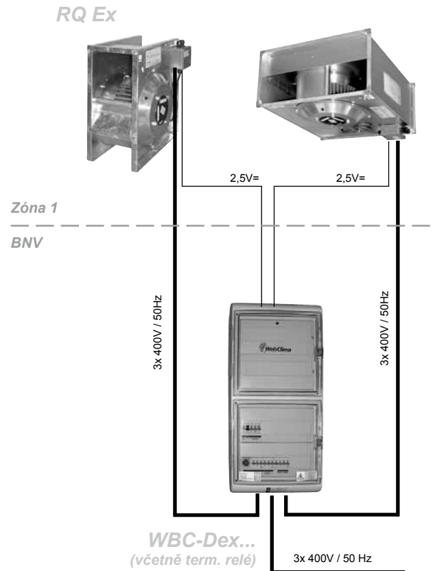
Obrázek 19 – zapojení ventilátoru
