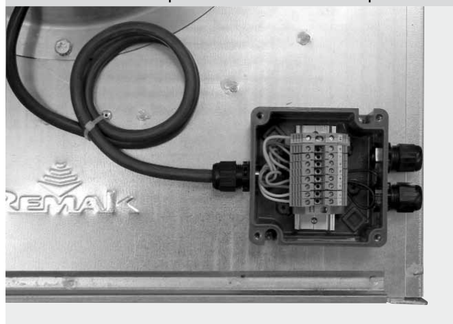
Obrázek 14 – celoplastová svorkovnice na plášti
