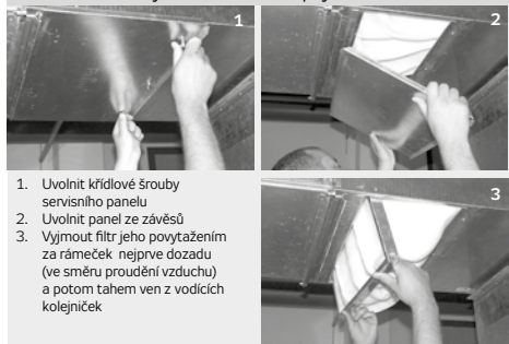
Obrázek 59 – výměna filtrační kapsy
