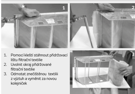
Obrázek 61 – výměna filtrační textilie
