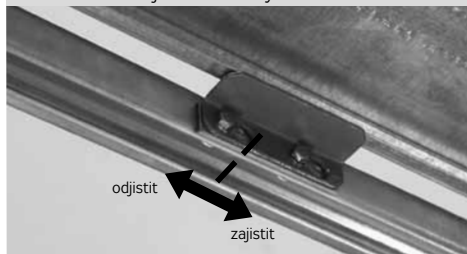
Obrázek 53 – zajišťovací šrouby
