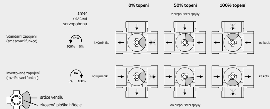
Obrázek 48 – funkce třicestného ventilu
