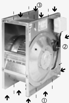
Obrázek 5 – kotevní otvory
