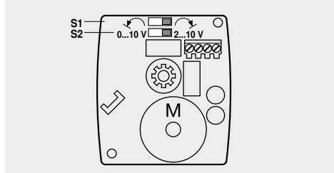
Obrázek 47 – přepínání směru otáčení servopohonu
