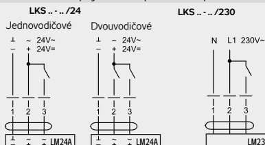
Obrázek 64 – Připojení servopohonů klapky
