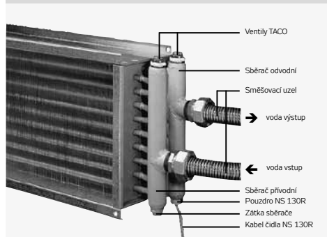
Obrázek 29 – instalace ventilu TACO
