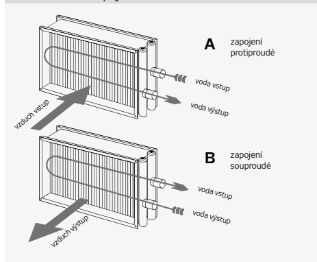
Obrázek 31 – zapojení ohřívače
