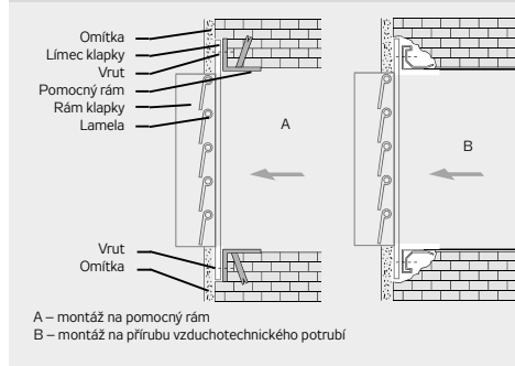
Obrázek 75 – montáž přetlakové klapky PK
