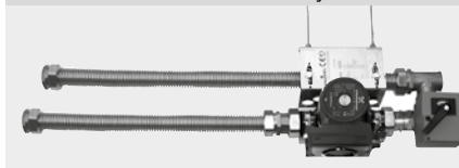
Obrázek 35 – montáž na závěsné tyče
