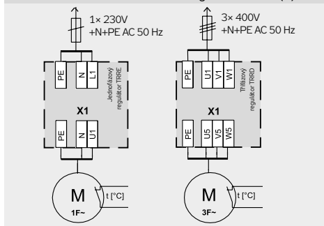
Obrázek 22 – svorkové schéma regulátorů TRRE(D)
