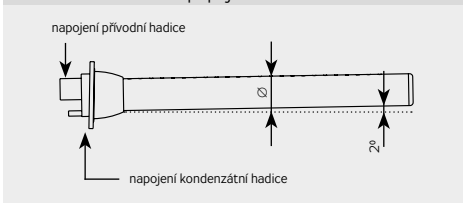
Obrázek 85 – sklon a připojení distribuční trubice
