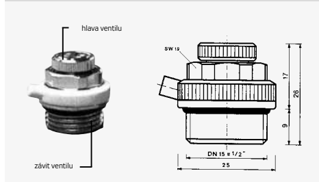
Obrázek 27 – odvodu vzdušňovací ventil TACO
