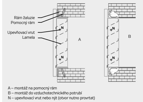
Obrázek 77 – montáž protidešťové žaluzie PZ
