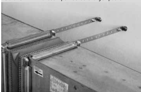
Obrázek 14 – zavěšení pomocí děrovaných pásů
