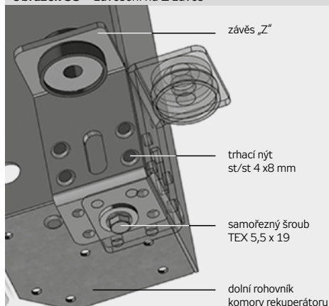
Obrázek 55 – zavěšení na Z závěs
