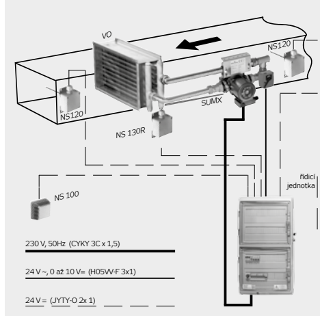
Obrázek 46 – připojení směšovacího uzlu
