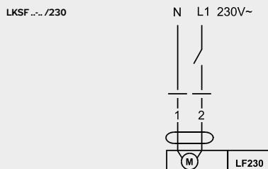
Obrázek 68 – Připojení servopohonu
