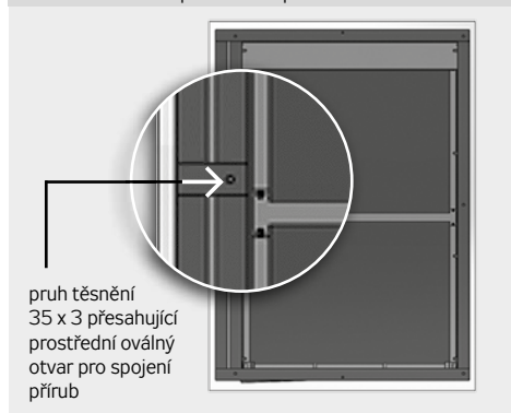
Obrázek 56 – nalepení samolepícího těsnění
