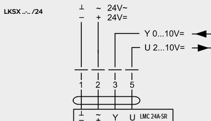
Obrázek 66 – Připojení servopohonu
