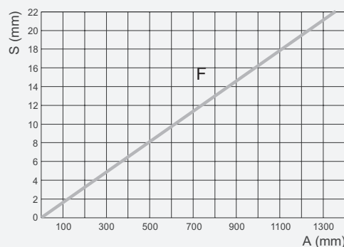
Abbildung 15 - Abgleich der Riemenscheiben
