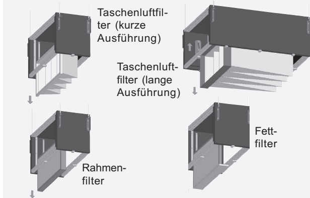
Abbildung 17 - Austausch der Filtereinlage
