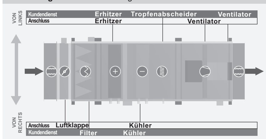
Abbildung 1 – Seitenausführung der Einheiten
