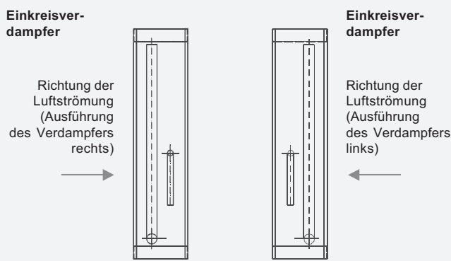
Abbildung 10 - Anschluss der Verdampfer
