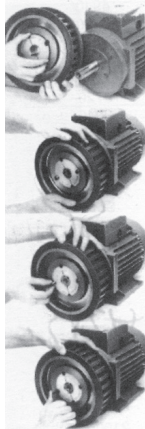
Abbildung 16 - Spannfutter Taper Lock®
