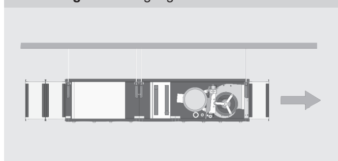
Abbildung 2 - Aufhängung unter der Decke
