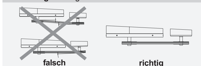
Abbildung 15 - Abgleich der Riemenscheiben
