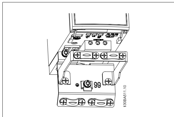
Ábra 3.5: VLT Micro Drive tehermentesítő kerettel
