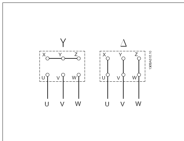
Ábra 3.3: Csillag- és háromszöghozkapcsolás
