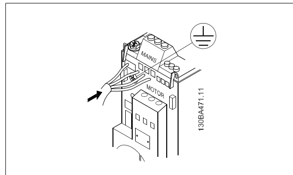
Ábra 3.1: A földelőkábel és a hálózati vezetékek csatlakoztatása
