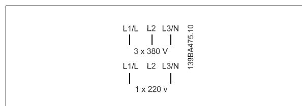
Ábra 3.2: A vezetékek háromfázisú és egyfázisú bekötése
