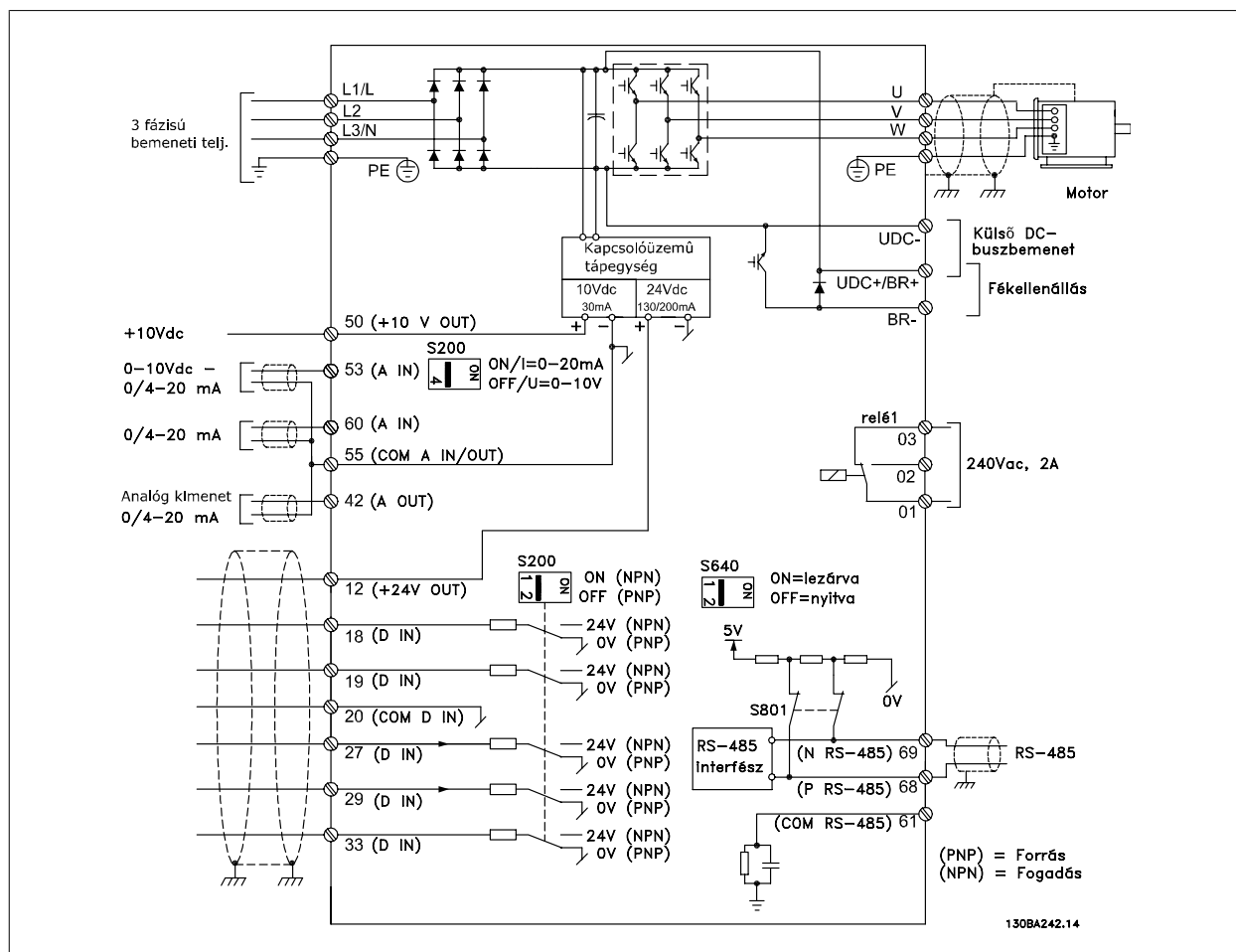
Ábra 3.10: Az összes villamos csatlakozót tartalmazó rajz
