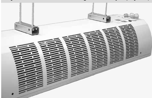
Rysunek 10 - montaż na gwintowanym pręcie (C1)
