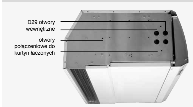
Rysunek 33 – Punkty łączące, D2
