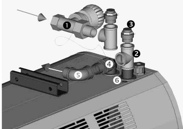
Rysunek 15 – podłączenie zaworu termostatycznego
