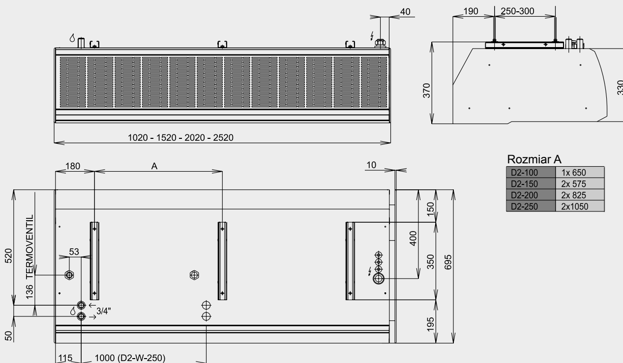
Rysunek 7 - podstawowe wymiary kurtyn typ D2
