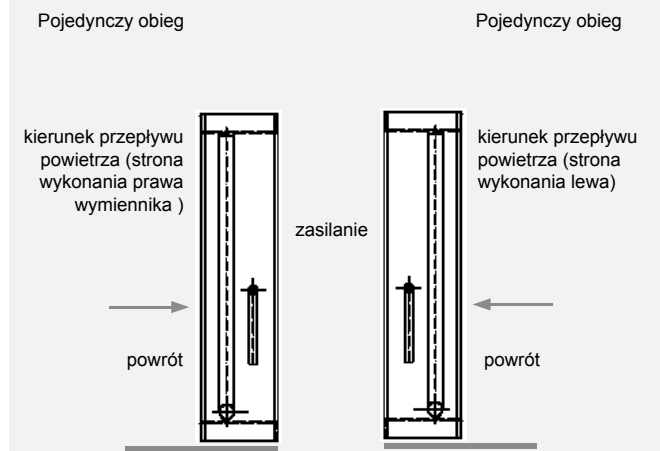
Rysunek 10 - podłączenie chłodziw z bezpośrednim odparowaniem
