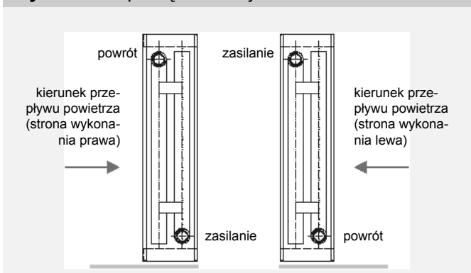
Rysunek 9 - podłączenie wymiennika
