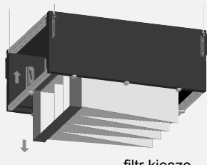
Rysunek 17 - wymiana wkładów filtrów
