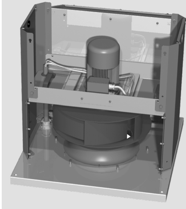
Rysunek 8 – prowadzenie kabli przez otwór
