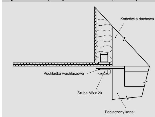
Rysunek 13 – podłączenie kanału do podstawy
