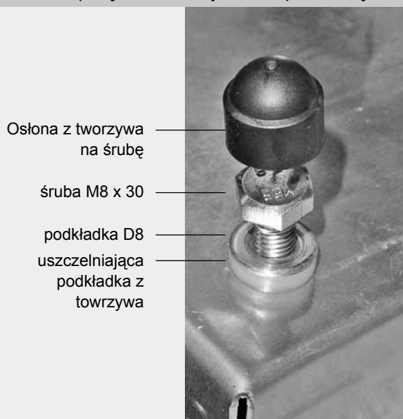
Rysunek 3 – połączenie wentylatora z podstawą
