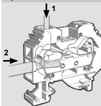
Rysunek 4 – Zacisk WAGO
