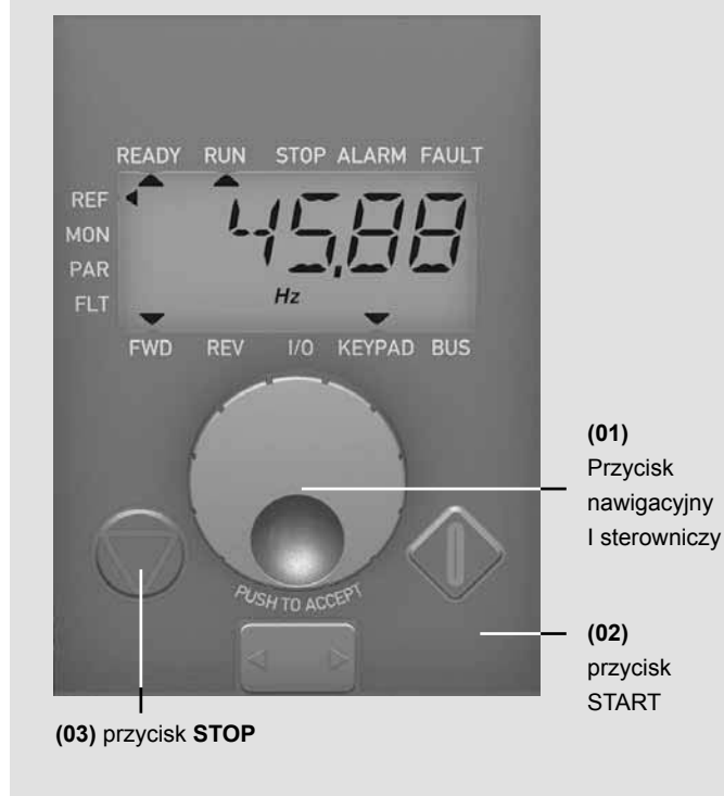
Rysunek 12 – panel sterowniczy
