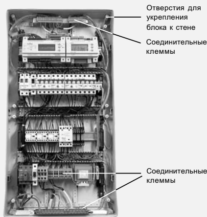
Рис. 8 – силовая часть блока VCB
