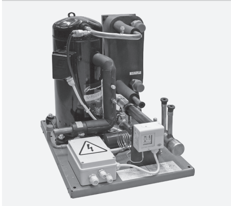
Obrázek 1 – sekce s vestavbou integrovaného chlazení
