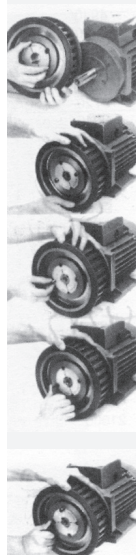
Obrázek 25 – upínací pouzdro Taper-Lock®
