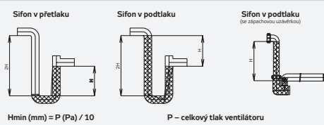
Obrázek 20 – odvod kondenzátu
