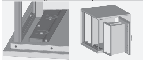
Obrázek 27 – vyjmutí filtrační vložky
