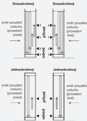
Obrázek 19 – zapojení výparníků
