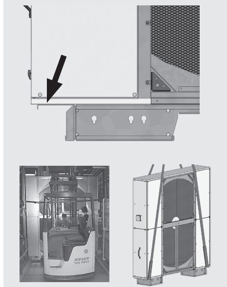
Рис 1 - Манипуляция с рекуператором
