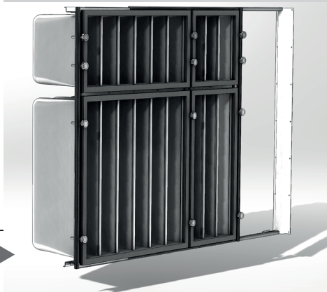
Рисунок 7 – Способ извлечения встроенного блока у XR 13 - XR 28
