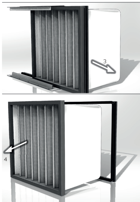
Рисунок 6 – Способ извлечения вставки с прочной рамой (XR04 – XR10)
