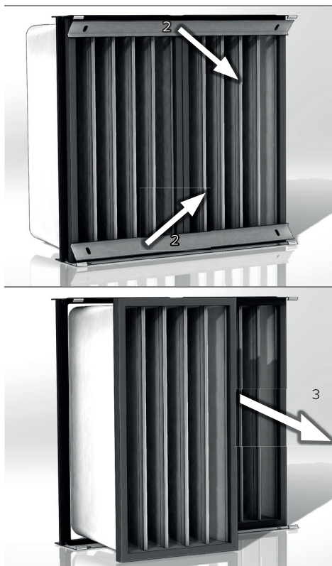
Рисунок 7 – Способ извлечения встроенного блока у XR 13 - XR 28
