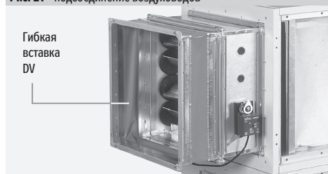
Рис. 21 – подсоединение воздухопроводов
