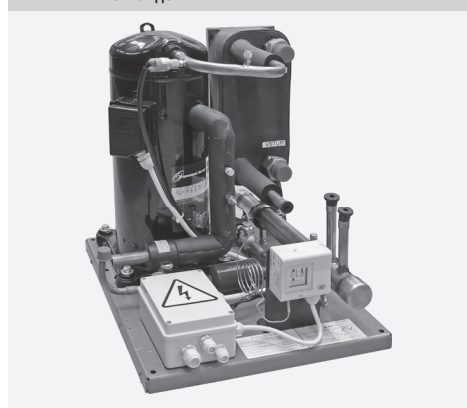
Рисунок 1 – Секция с встроенным блоком интегрированного охлаждения
