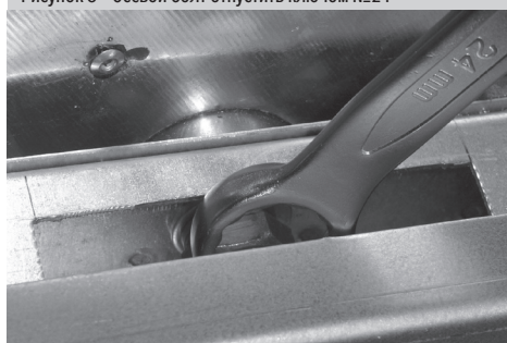
Рисунок 8 – Осевой болт отпустить ключом №24
