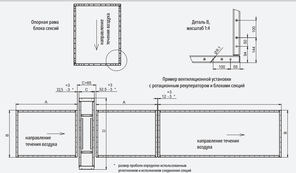
Рис. 5 – расположение опорной рамы
