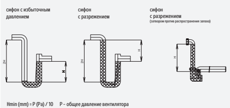
Рис. 20 – отвод конденсата
