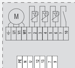
Рисунок 4 – Схема соединений регенератора
