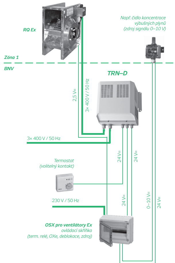
OBRÁZEK 16 – ZAPOJENÍ VENTILÁTORU
