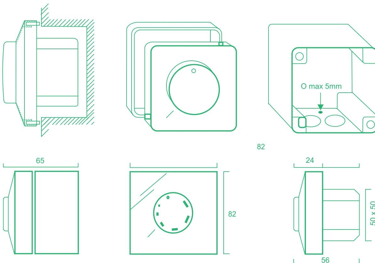
OBRÁZEK 48 – MONTÁŽNÍ INSTRUKCE
