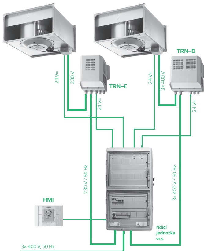
OBRÁZEK 23 – ZAPOJENÍ REGULÁTORŮ
