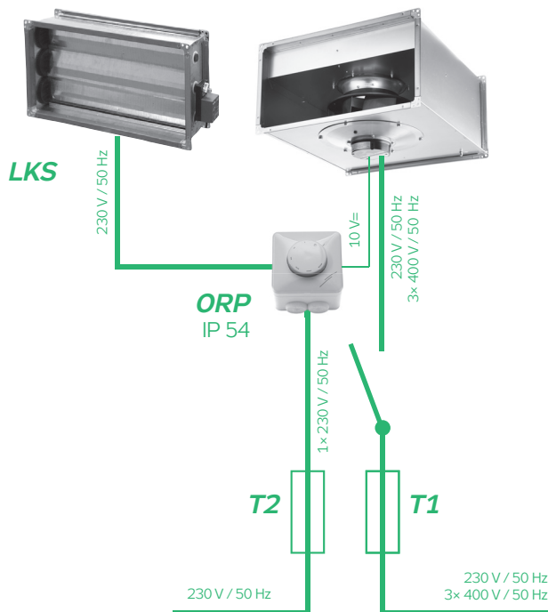
OBRÁZEK 45 – ZAHOJENÍ OVLADAČE
