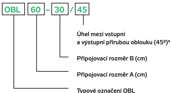
OBRÁZEK 9 – PŘÍKLAD OZNAČENÍ OBLOKU
