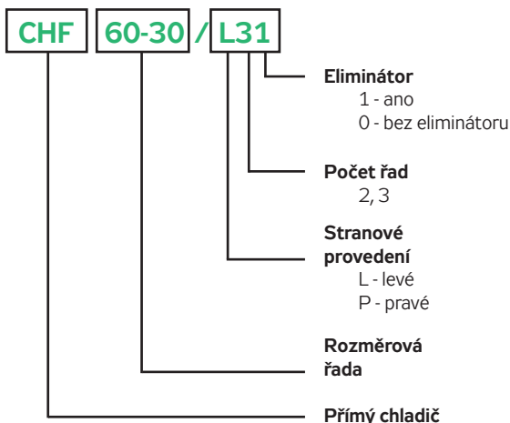
OBRÁZEK 2 – TYPOVÉ ZNAČENÍ
