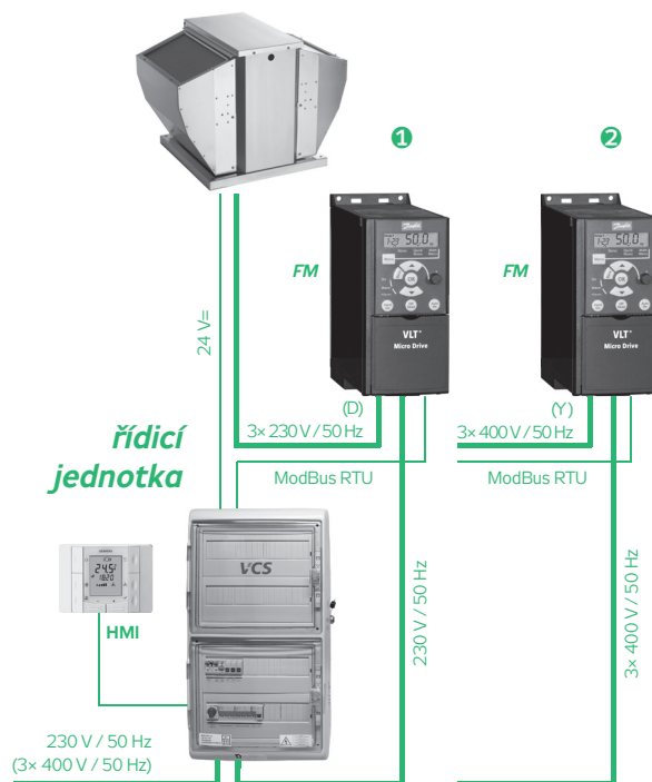
OBRÁZEK 12 – ZAPOJENÍ VENTILÁTORU
