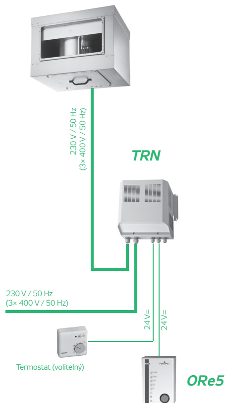
OBRÁZEK 7 – ZAPOJENÍ VENTILÁTORU
