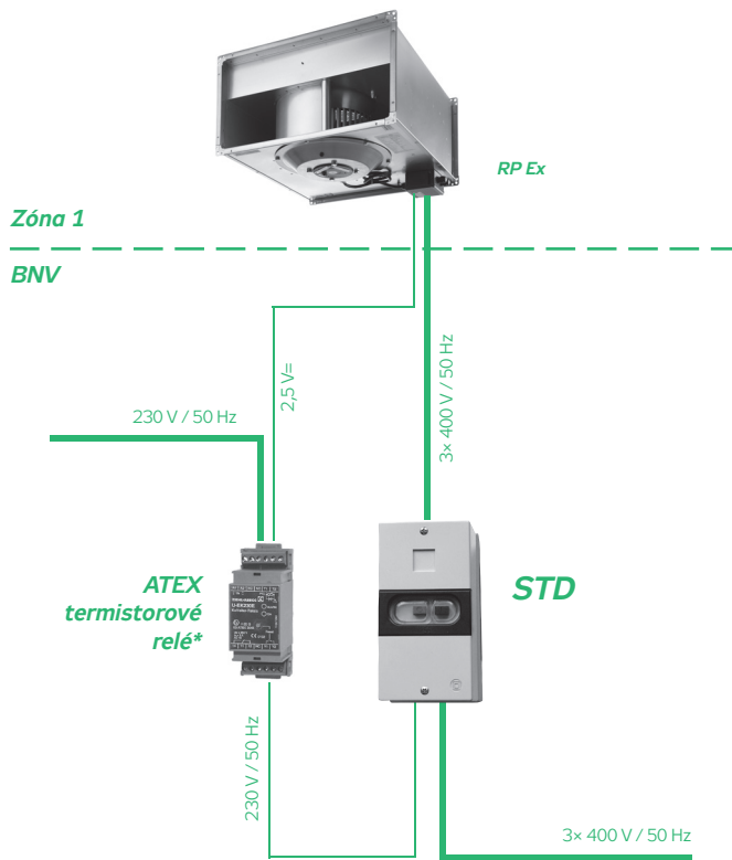
OBRÁZEK 12 – ZAPOJENÍ VENTILÁTORU
