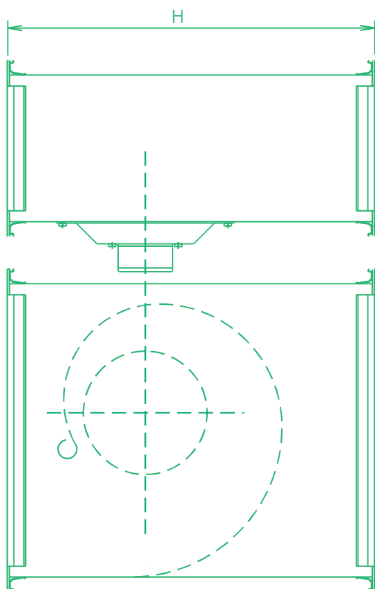
OBRÁZEK 5 – ROZMĚRY VENTILÁTORŮ
