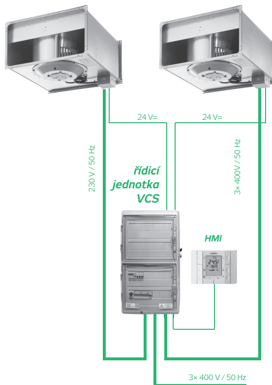
OBRÁZEK 9 – ZAPOJENÍ VENTILÁTORŮ
