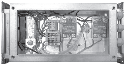
EOS... / 3, obsahují dvě jednofázové spínací relé SSR. Pohled do elektroinstalační skříňe ohřívače EOS 30-15/3 po odkrytí ochranného krytu.
