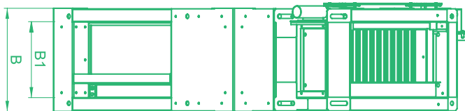
OBRÁZEK 4 – ROZMĚRY
