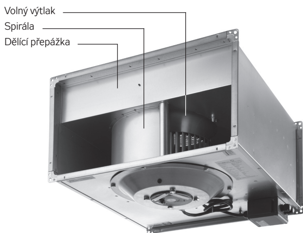
OBRÁZEK 6 – USPOŘÁDÁNÍ VÝTLAKU VENTILÁTORU RP EX
