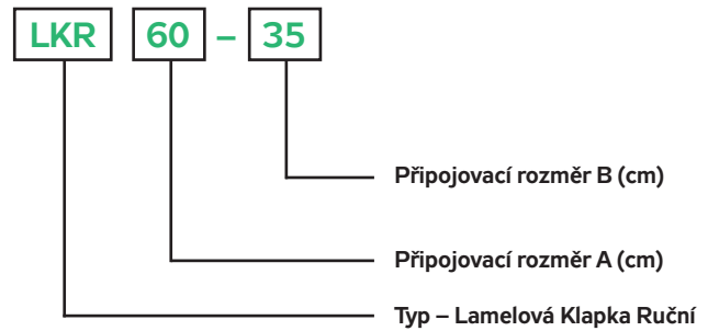
OBRÁZEK 2 – TYPOVÉ OZNAČENÍ
