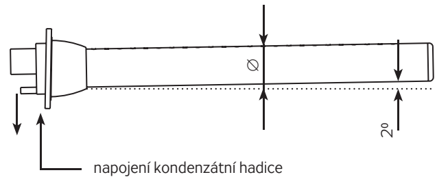
OBRÁZEK 3 – SKLON A PŘIPOJENÍ DISTRIBUČNÍ TRUBICE
