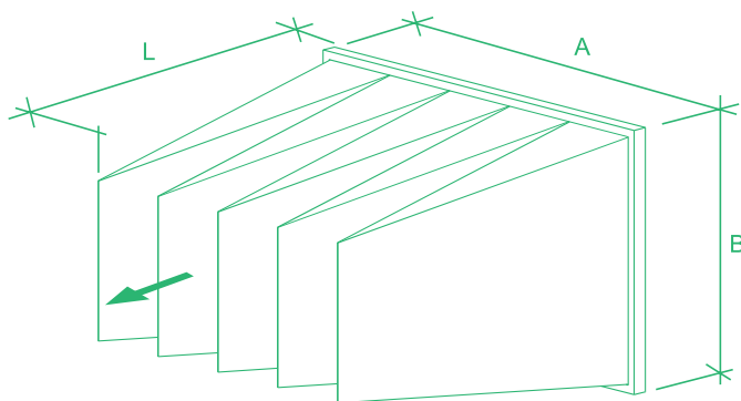
OBRÁZEK 2 – TYPOVÉ OZNAČENÍ
