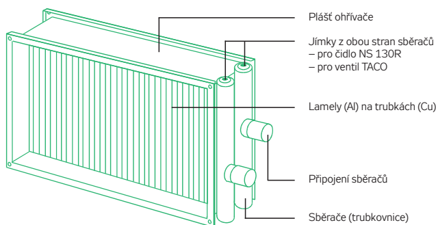
OBRÁZEK 2 – KONSTRUKCE OHŘÍVAČE
