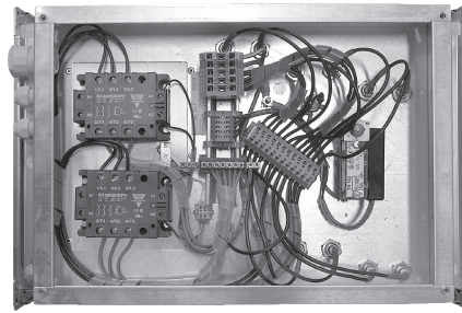
EOS... /22 – 45, EOSX .../12 – 45, (obsahují dvě nebo tři třífázové spínací relé SSR). Pohled do EOSX se dvěma sekcemi (resp. SSR).
