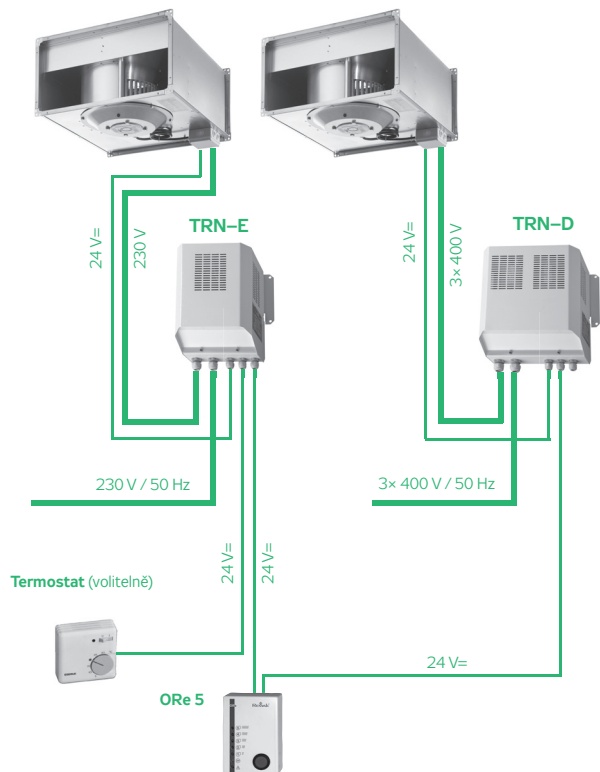
OBRÁZEK 22 – ZAPOJENÍ REGULÁTORŮ
