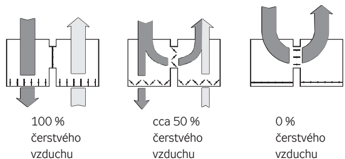
OBRÁZEK 4 – ZNÁZORNĚNÍ FUNKCE SMĚŠOVACÍ KOMORY SKX
