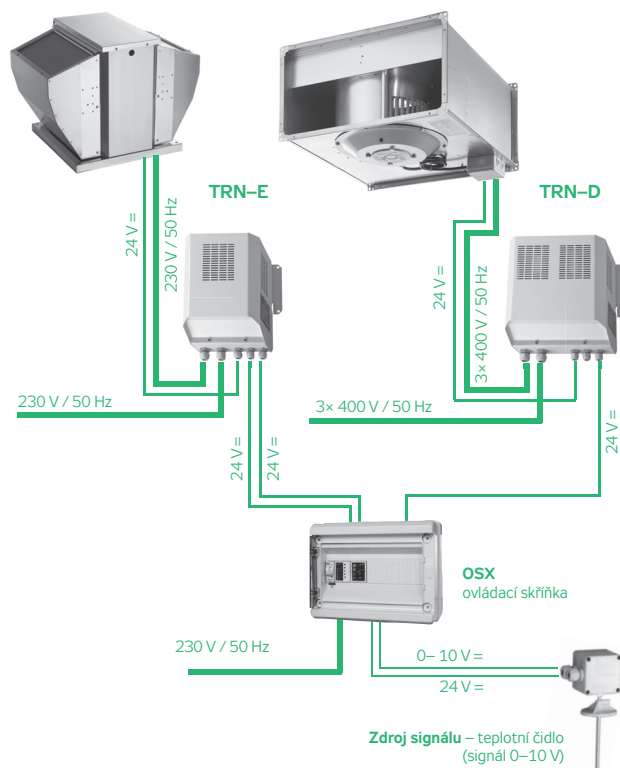
OBRÁZEK 24 – ZAPOJENÍ REGULÁTORŮ
