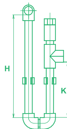
OBRÁZEK 5 – PŘÍKLAD SIFONU PRO ODVOD KONDENZÁTU
