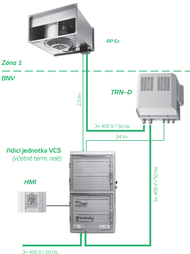
OBRÁZEK 15 – ZAPOJENÍ VENTILÁTORU
