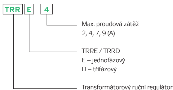
OBRÁZEK 29 – REGULÁTOR ŘADY TRRE(D)
