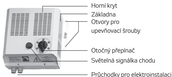
OBRÁZEK 30 – SLOŽENÍ REGULÁTORU
