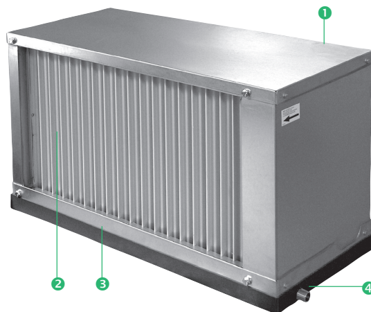
OBRÁZEK 2 – POPIS ČÁSTÍ ELIMINÁTORU KAPEK
