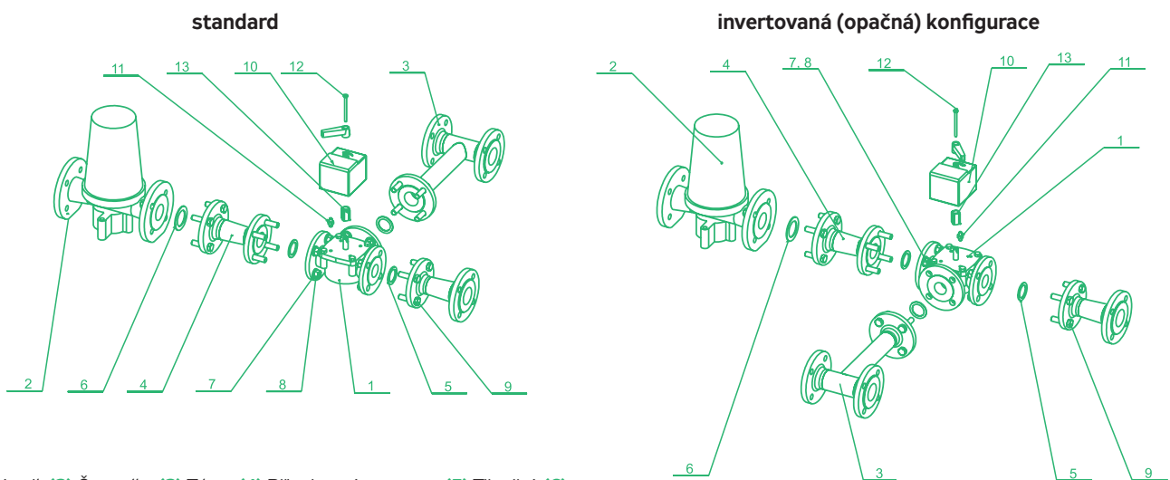
OBRÁZEK 7 – ROZKLAD PŘÍRUBOVÉHO UZLU
