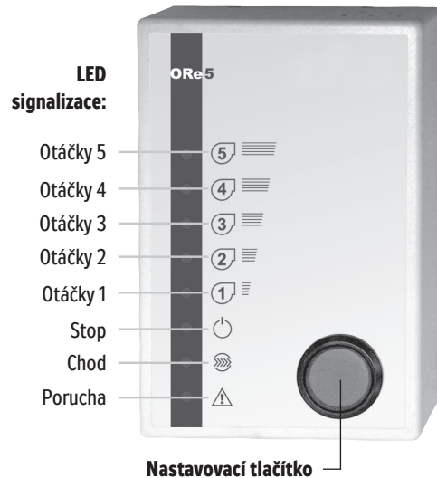
OBRÁZEK 25 – ČELNÍ PANEL
