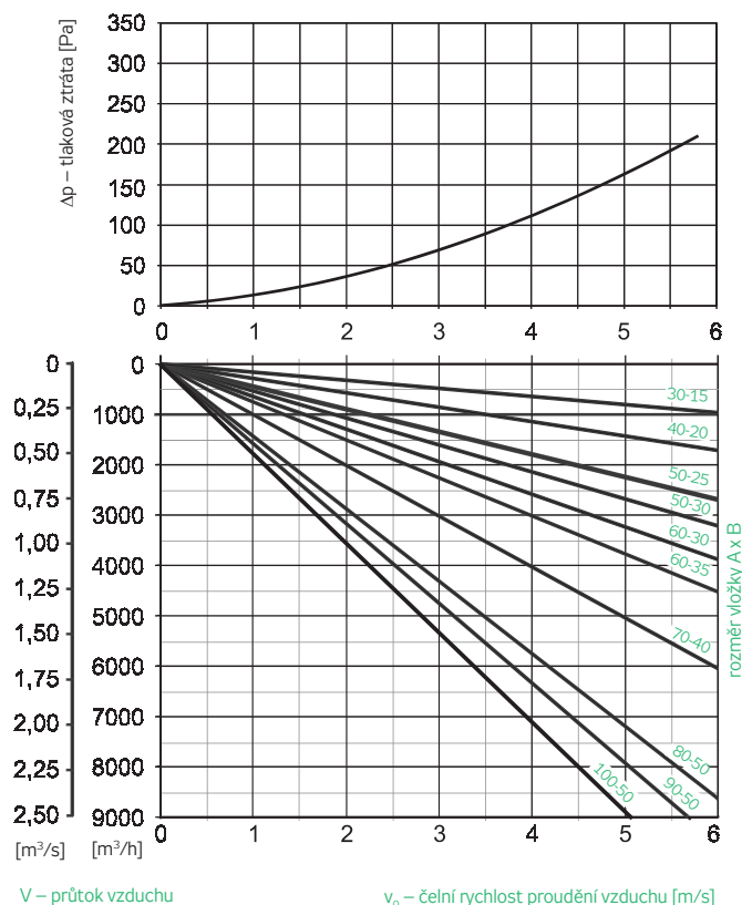
GRAF 1 – TLAKOVÁ ZTRÁTA VLOŽKOVÝCH FILTRŮ VFK V ČISTÉM STAVU
