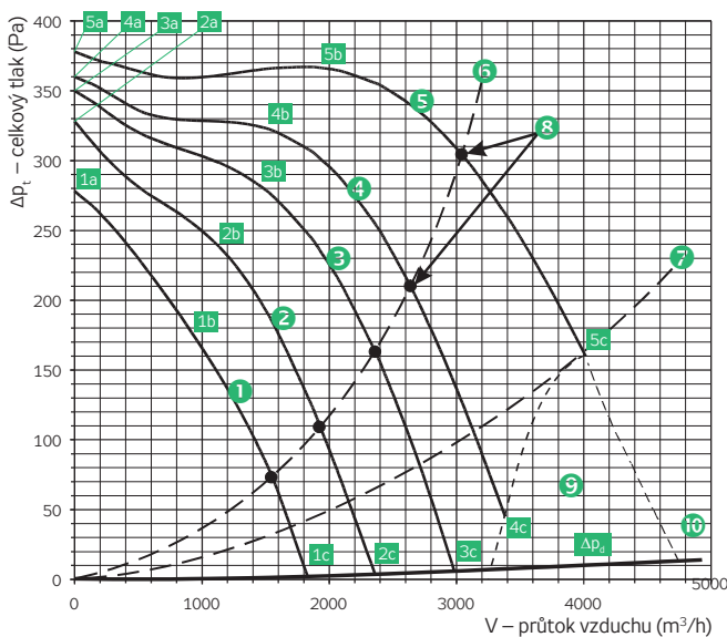
GRAF 1 – PRACOVNÍ KŘIVKY VÝSTUPNÍHO NAPĚTÍ
