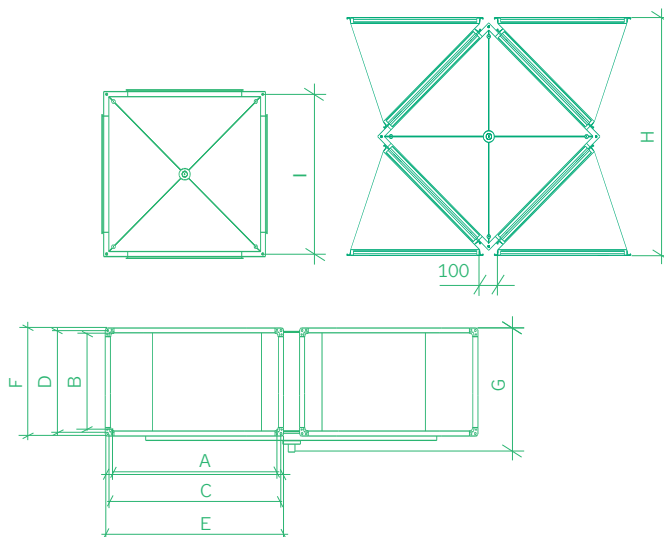
OBRÁZEK 4 – ROZMĚRY REKUPERÁTORŮ
