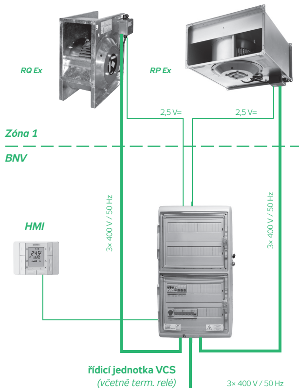
OBRÁZEK 14 – ZAPOJENÍ VENTILÁTORU
