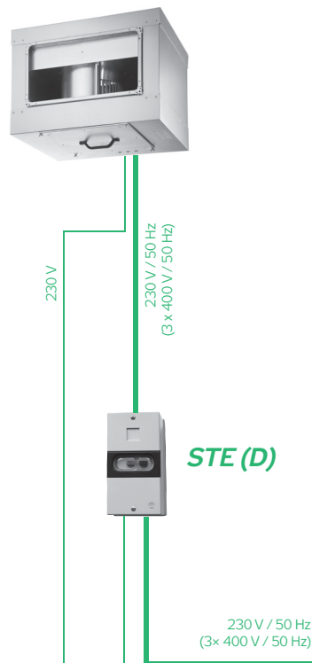
OBRÁZEK 6 – ZAPOJENÍ VENTILÁTORU
