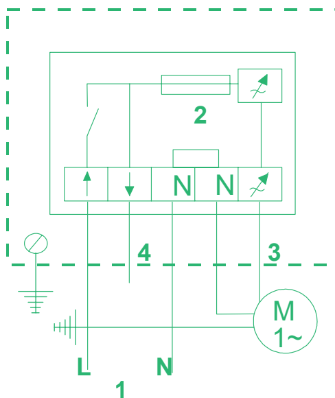
OBRÁZEK 49 – EL. ZAPOJENÍ REGULÁTORU
