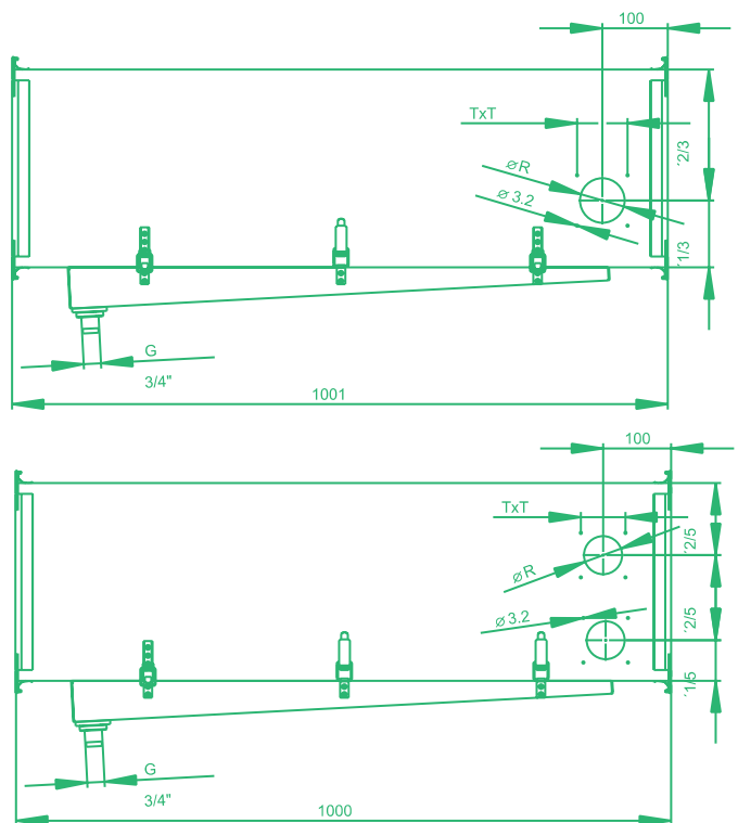
OBRÁZEK 1 – ROZMĚRY KOMOR ZVLHČOVAČE
