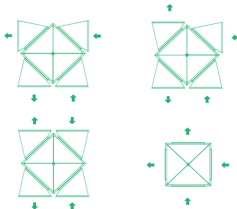
OBRÁZEK 6 – VARIANTY DISPOZIČNÍHO USPOŘÁDÁNÍ V POTRUBÍ PODLE ORIENTACE OBLOUKŮ OBL ... /45
