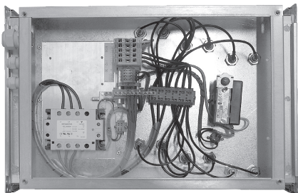
OBRÁZEK 12 – SKŘÍŇ OHŘÍVAČE EOS PO ODKRYTÍ KRYTU
