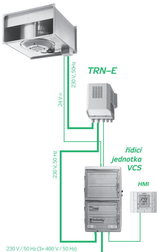
OBRÁZEK 10 – ZAPOJENÍ VENTILÁTORU
