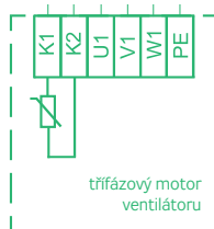
OBRÁZEK 11 – SCHÉMA ZAPOJENÍ
