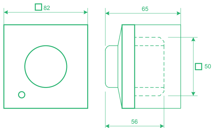
OBRÁZEK 47 – ROZMĚRY REGULÁTORU
