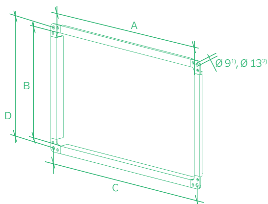
OBR. 1 – ROZMĚROVÁ ŘADA
