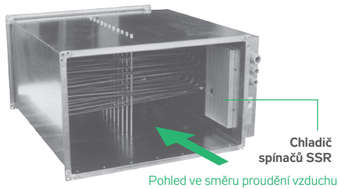
OBRÁZEK 9 – UMÍSTĚNÍ CHLADIČE SPÍNAČŮ
