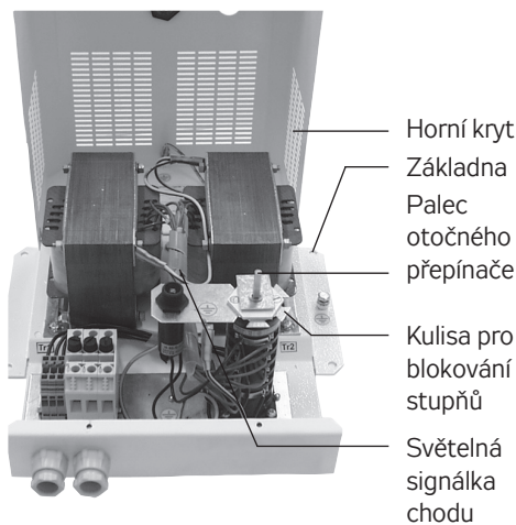
OBRÁZEK 33 – MECHANICKÉ BLOKOVÁNÍ
