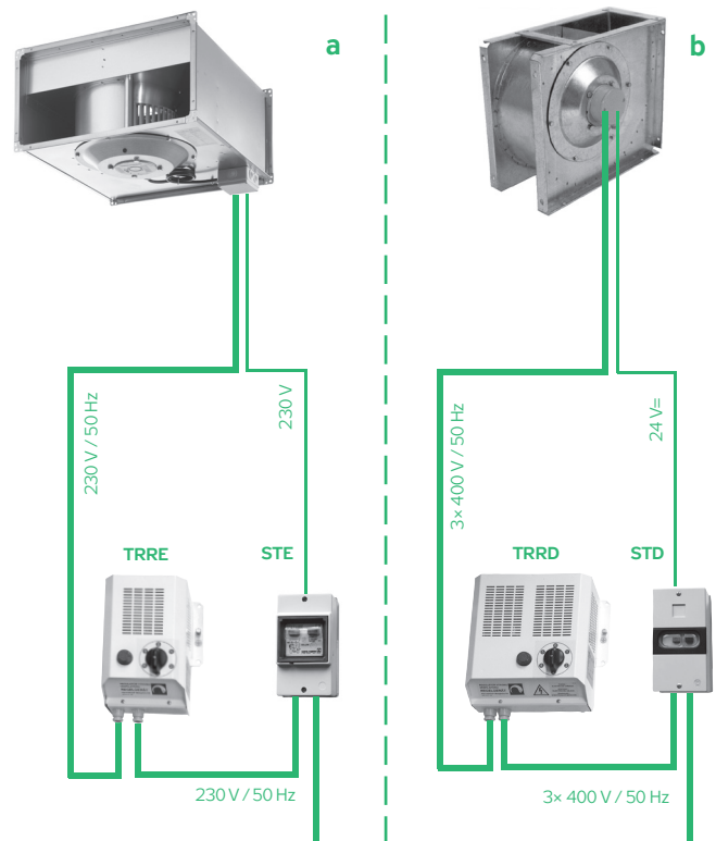
OBRÁZEK 35 – ZAPOJENÍ REGULÁTORŮ
