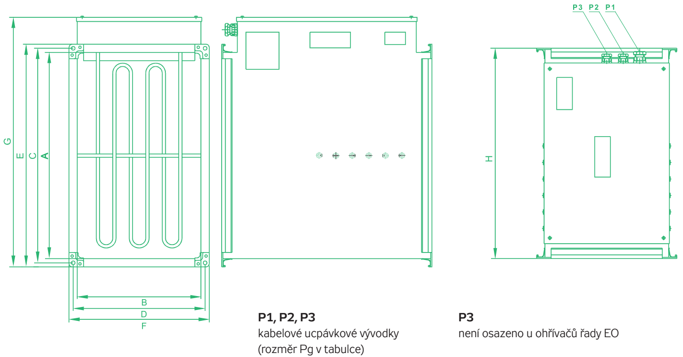
OBRÁZEK 3 – ROZMĚRY A HMOTNOSTI
