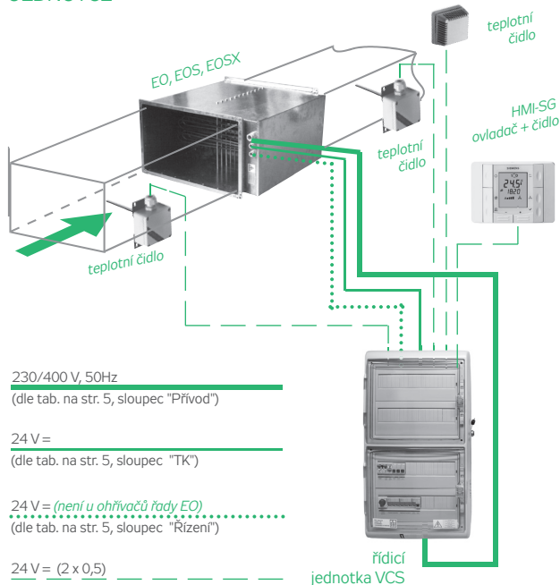
OBRÁZEK 6 PŘÍKLAD PŘIPOJENÍ OHŘÍVAČŮ K ŘÍDICÍ JEDNOTCE
