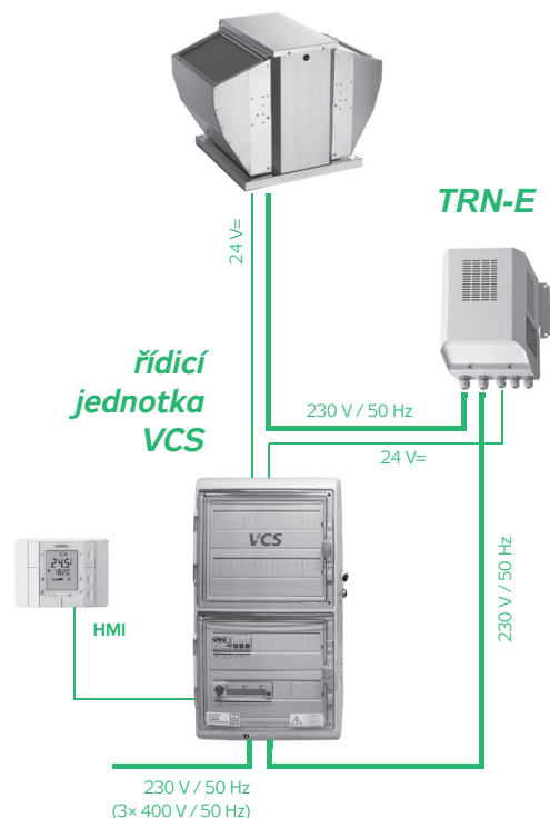
OBRÁZEK 11 – ZAPOJENÍ VENTILÁTORU
