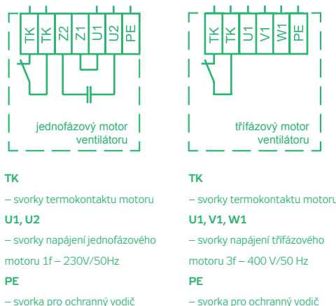
OBRÁZEK 5 – SCHÉMATA ZAPOJENÍ
