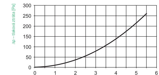
GRAF 1 – TLAKOVÁ ZTRÁTA FILTRŮ FT V ČISTÉM STAVU
