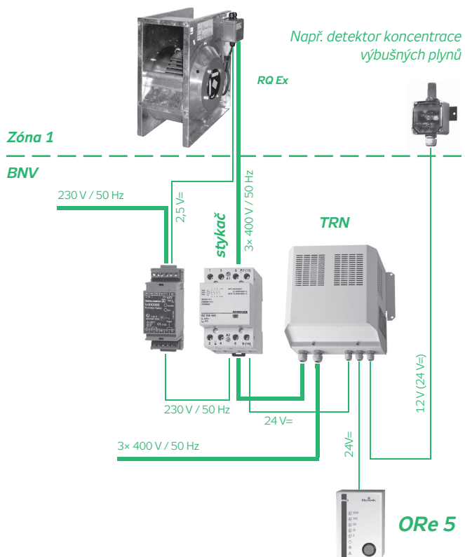
OBRÁZEK 13 – ZAPOJENÍ VENTILÁTORU
