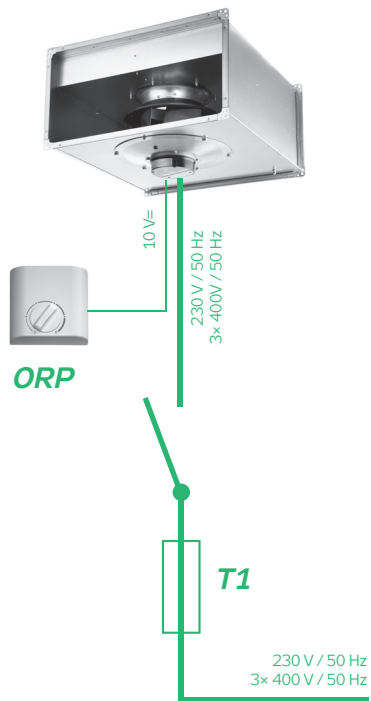
OBRÁZEK 44 – ZAHOJENÍ OVLADAČE
