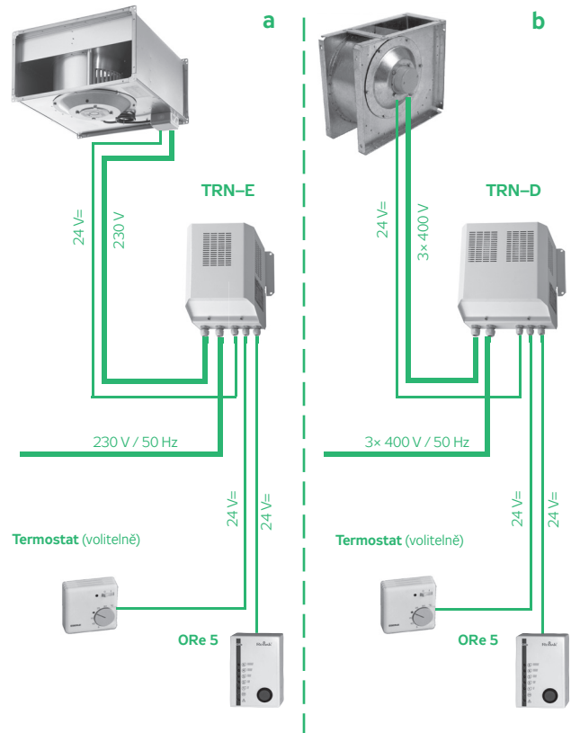
OBRÁZEK 21 – ZAPOJENÍ REGULÁTORŮ
