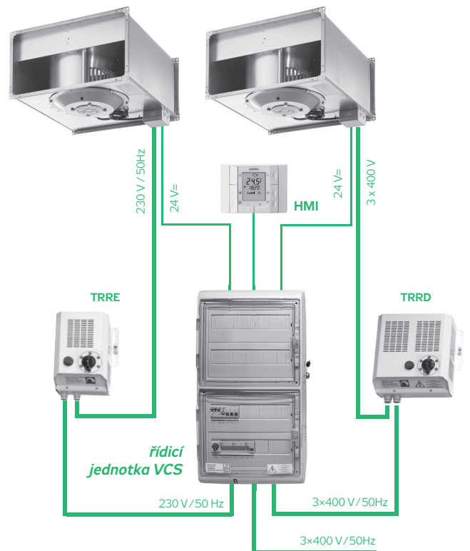
OBRÁZEK 36 – ZAPOJENÍ REGULÁTORŮ
