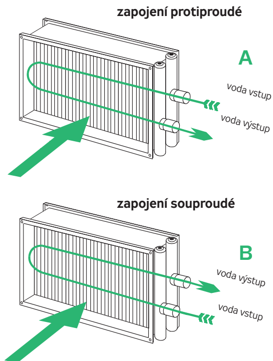
OBRÁZEK 8 – ZAPOJENÍ OHŘÍVAČE
