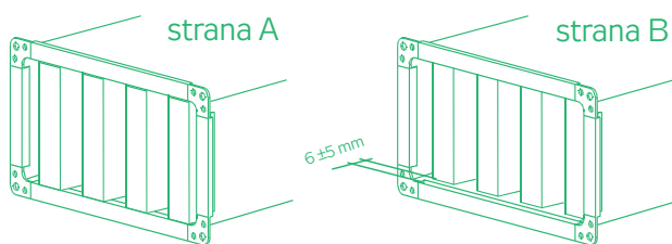
OBRÁZEK 3 – ORIENTACE TLUMIČŮ PŘI JEJICH SPOJOVÁNÍ
