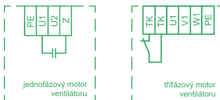
OBRÁZEK 4 – SCHÉMA ZAPOJENÍ
