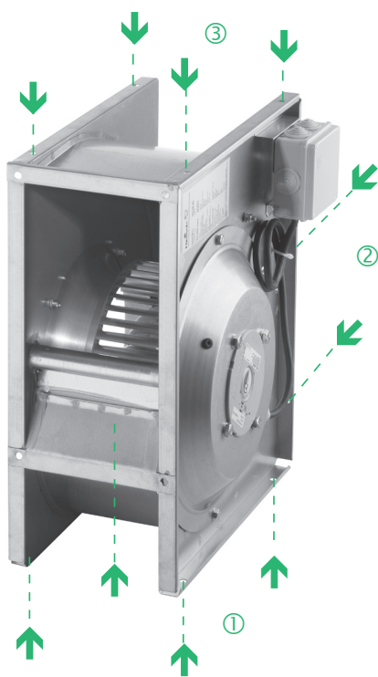
OBRÁZEK 3 – KOTEVNÍ OTVORY
