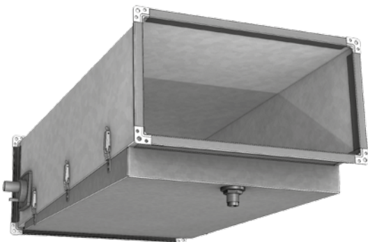
OBRÁZEK 2 – SESTAVENÁ KOMORA A ODVOD ONDENZÁTU
