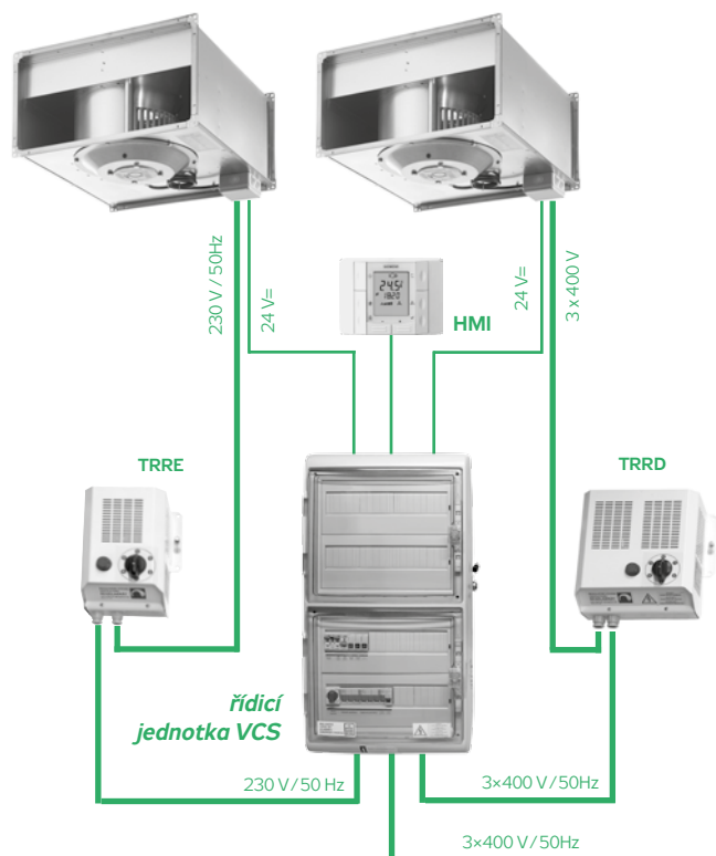
OBRÁZEK 36 – ZAPOJENÍ REGULÁTORŮ
