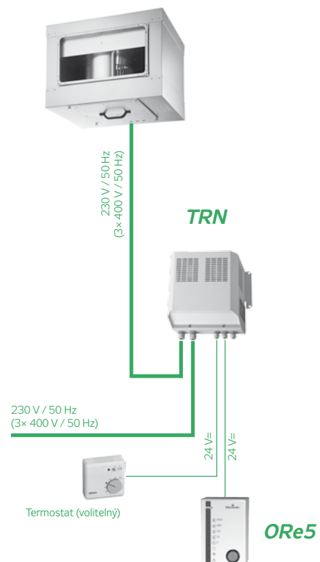
OBRÁZEK 7 – ZAPOJENÍ VENTILÁTORU
