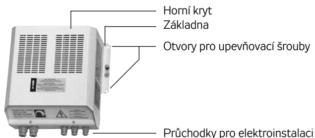
OBRÁZEK 17 – SLOŽENÍ REGULÁTORU
