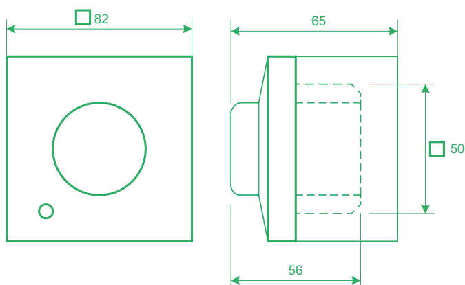
OBRÁZEK 47 – ROZMĚRY REGULÁTORU
