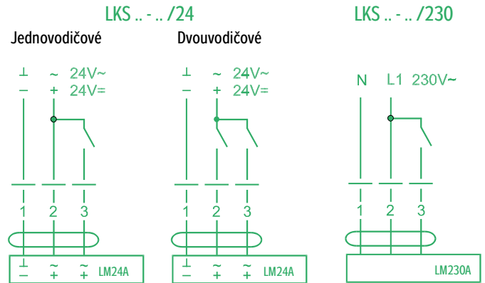
OBRÁZEK 4 – PŘIPOJENÍ SERVOPOHONŮ KLAPEK
