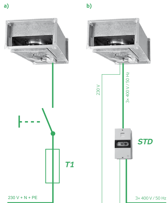
OBRÁZEK 5 – ZAPOJENÍ VENTILÁTORU
