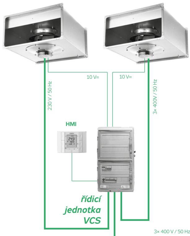
OBRÁZEK 8 – ZAPOJENÍ VENTILÁTORU
