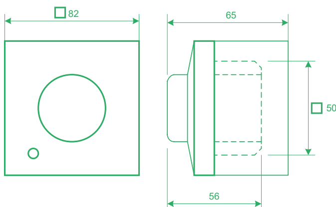
OBRÁZEK 47 – ROZMĚRY REGULÁTORU
