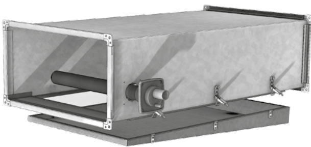
OBRÁZEK 2 – SESTAVENÁ KOMORA A ODVOD ONDENZÁTU
