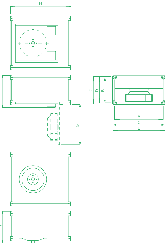
OBRÁZEK 5 – ROZMĚRY VENTILÁTORŮ
