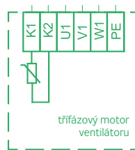
OBRÁZEK 10 – SCHÉMA ZAPOJENÍ
