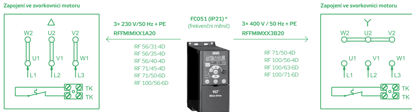
OBRÁZEK 3 – ZAPOJENÍ Y/Δ NA SVORKOVNICI 3F MOTORU S FREKVENČNÍM MĚNIČEM FC051 (IP21) – RFFMIMXXXX20
