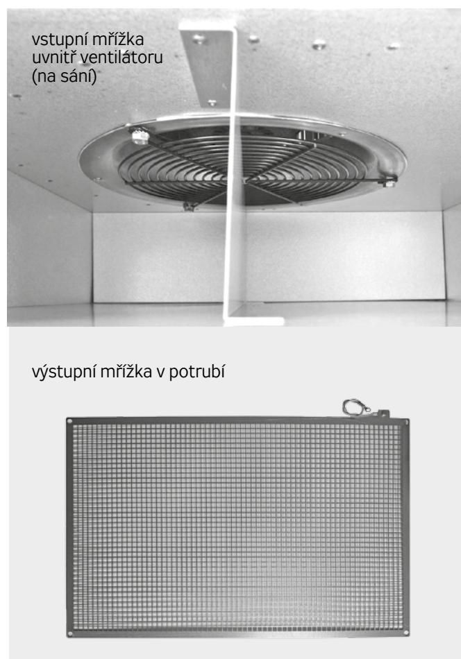
OBRÁZEK 8 – PŘÍKLAD PŘIHOVĚŘENÍ OCHRANNÉ MŘÍŽKY
