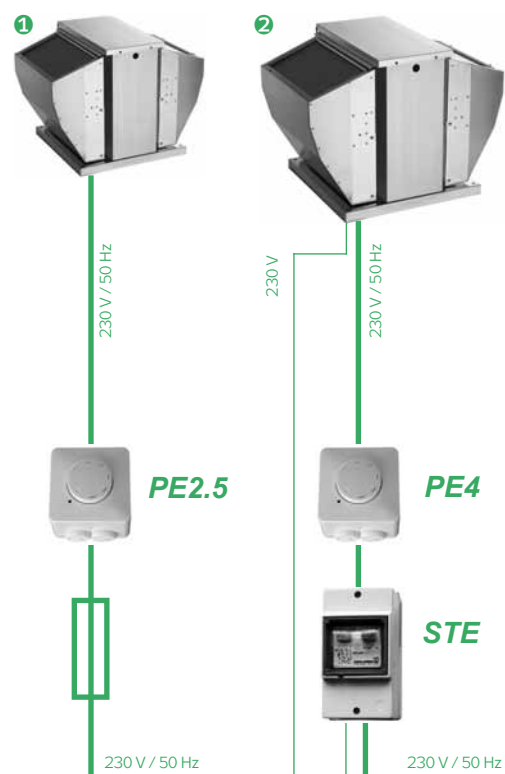
OBRÁZEK 7 – ZAPOJENÍ VENTILÁTORU
