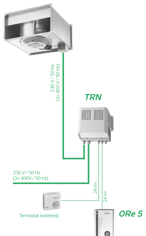
OBRÁZEK 8 – ZAPOJENÍ VENTILÁTORU
