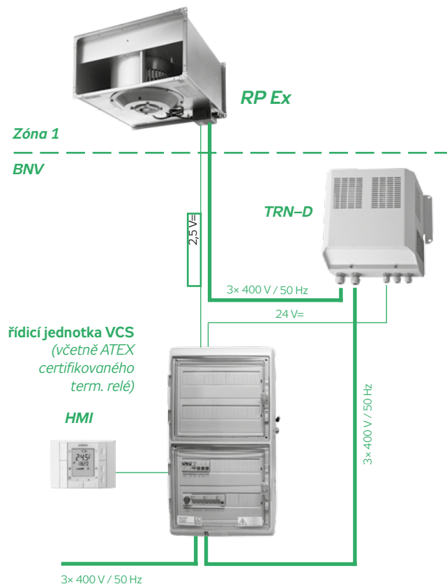
OBRÁZEK 14 – ZAPOJENÍ VENTILÁTORU
