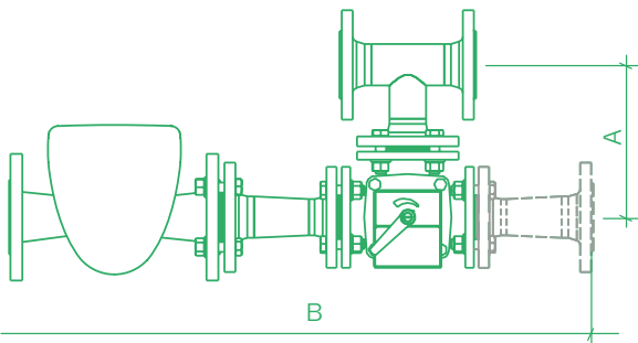
OBRÁZEK 4B – ZÁKLADNÍ DISPOZICE
