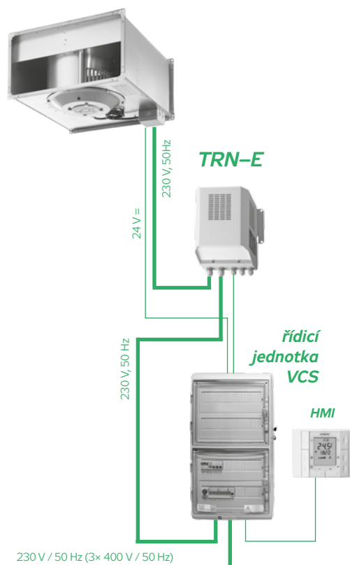
OBRÁZEK 10 – ZAPOJENÍ VENTILÁTORU
