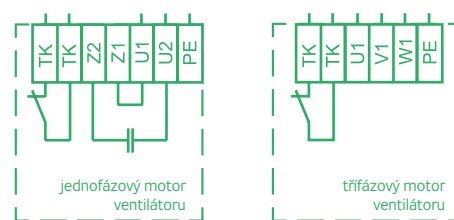
OBRÁZEK 6 – SCHÉMATA ZAPOJENÍ
