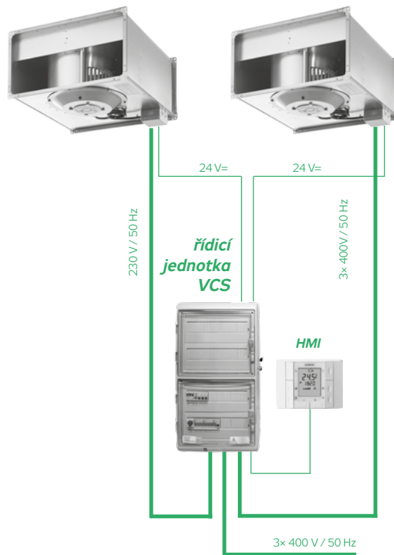
OBRÁZEK 9 – ZAPOJENÍ VENTILÁTORŮ
