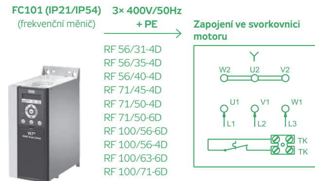
OBRÁZEK 4 – ZAPOJENÍ Y/Δ NA SVORKOVNICI 3F MOTORU S FREKVENČNÍM MĚNIČEM FC101 (IP21/IP54) – RFFMIBXX3B20 / RFFMIBXX3B50
