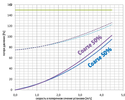
Исходная потеря давления карманного фильтра Coarse 50% и Coarse 60%
