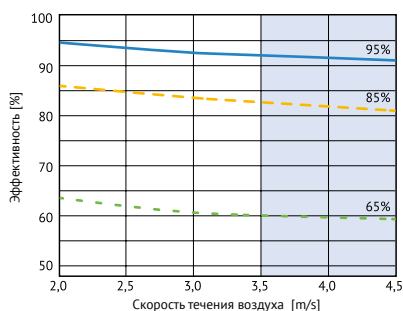
Эффективность увлажнения
