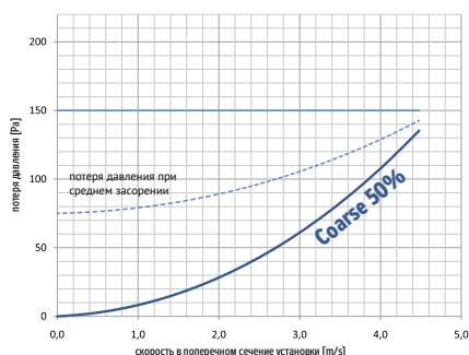
Исходная потеря давления жирового фильтра
