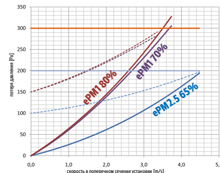
Исходная потеря давления карманного фильтра ePM2.5 65%, ePM1 70% и ePM1 80%
