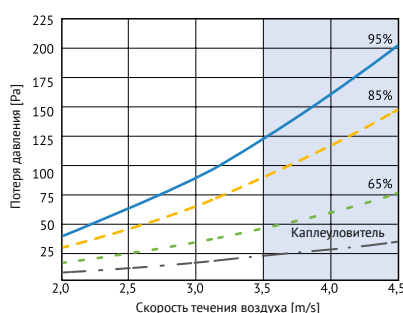
Потеря давления
