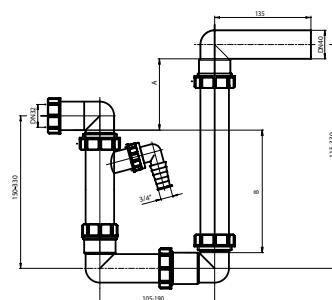
Сифон, предварительно заполняемый водой
