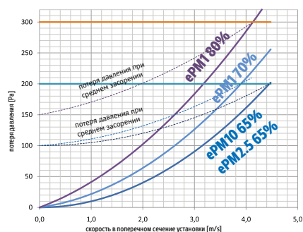
Исходная потеря давления компактных фильтров
