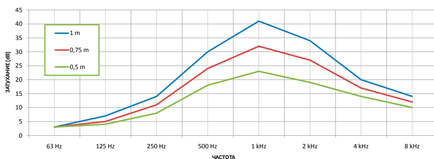
Затухание шумоглушителей
