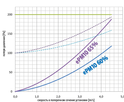
Исходная потеря давления карманного фильтра ePM10 60%, ePM10 65%
