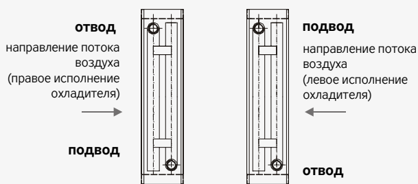
Рис. 18 – подсоединение испарителей
