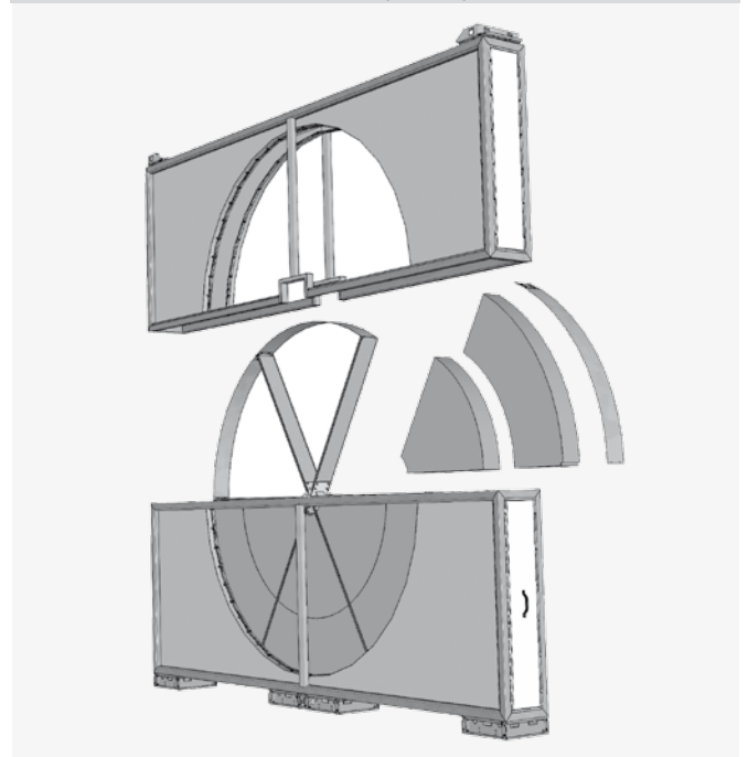
Рис. 13 – теплообменник в разобранном виде
