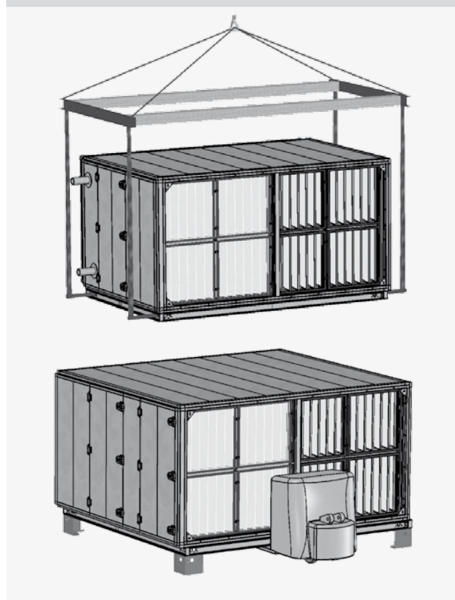
Рис. 2 – варианты подъема
