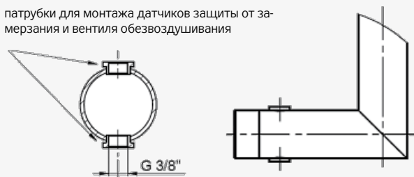
Рис. 17 – монтажа датчиков защиты от замерзания
