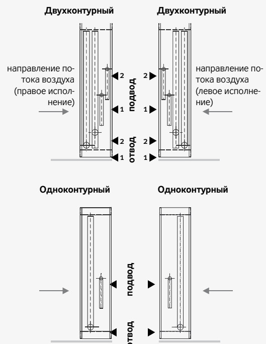
Рис. 20 – прямые испарители
