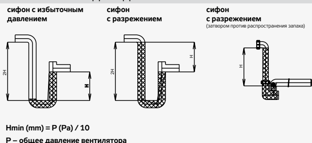
Рис. 21 – отвод конденсата
