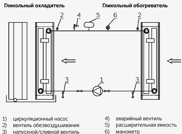
Рис. 19 – подключение гликолевого контура
