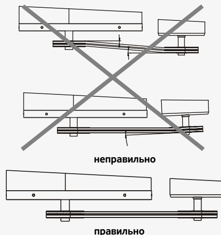
Рис. 26 – выравнивание шкивов
