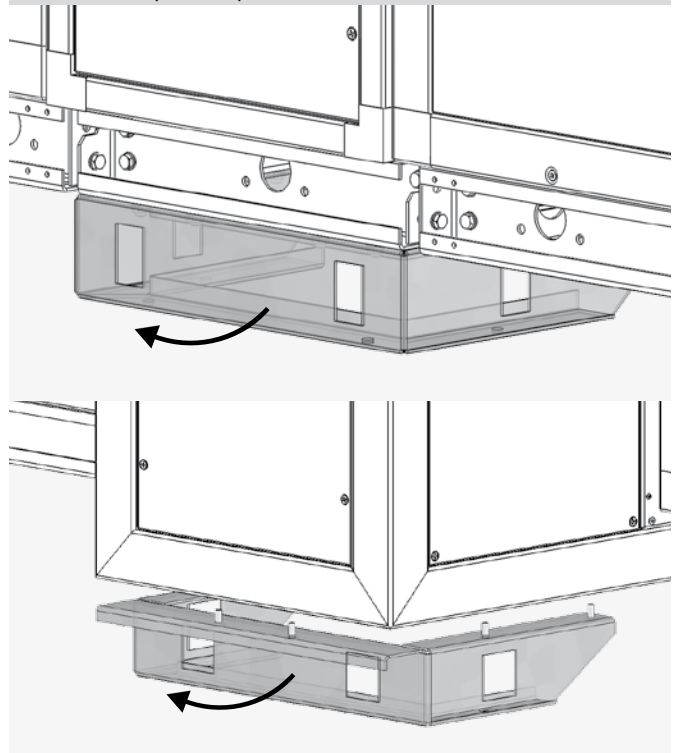
Рис. 12 – транспортные ножки
