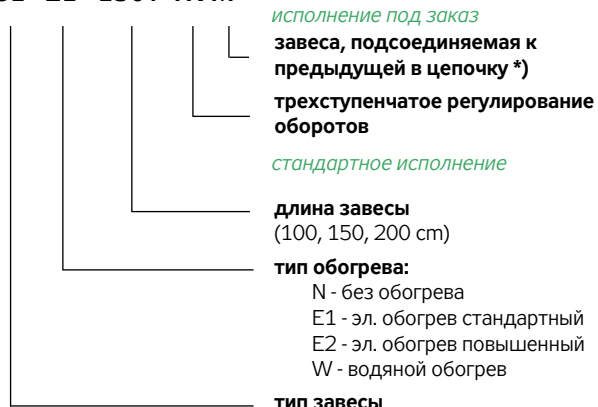
РИС. 4 – ОБОЗНАЧЕНИЕ ЗАВЕС СЕРИИ C1
