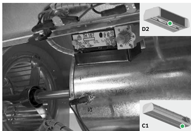
РИС. 13 – РЕГУЛИРУЮЩИЙ ТЕРМОСТАТ TH167
