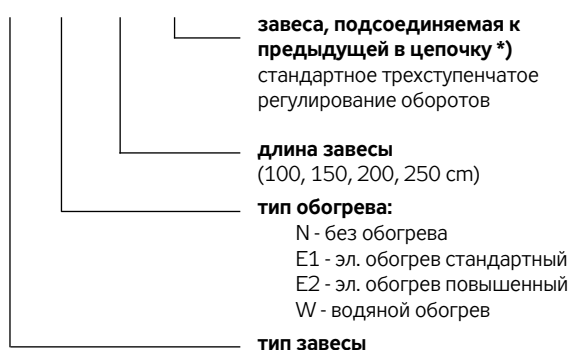
РИС. 10 – ОБОЗНАЧЕНИЕ ЗАВЕС СЕРИИ D2
