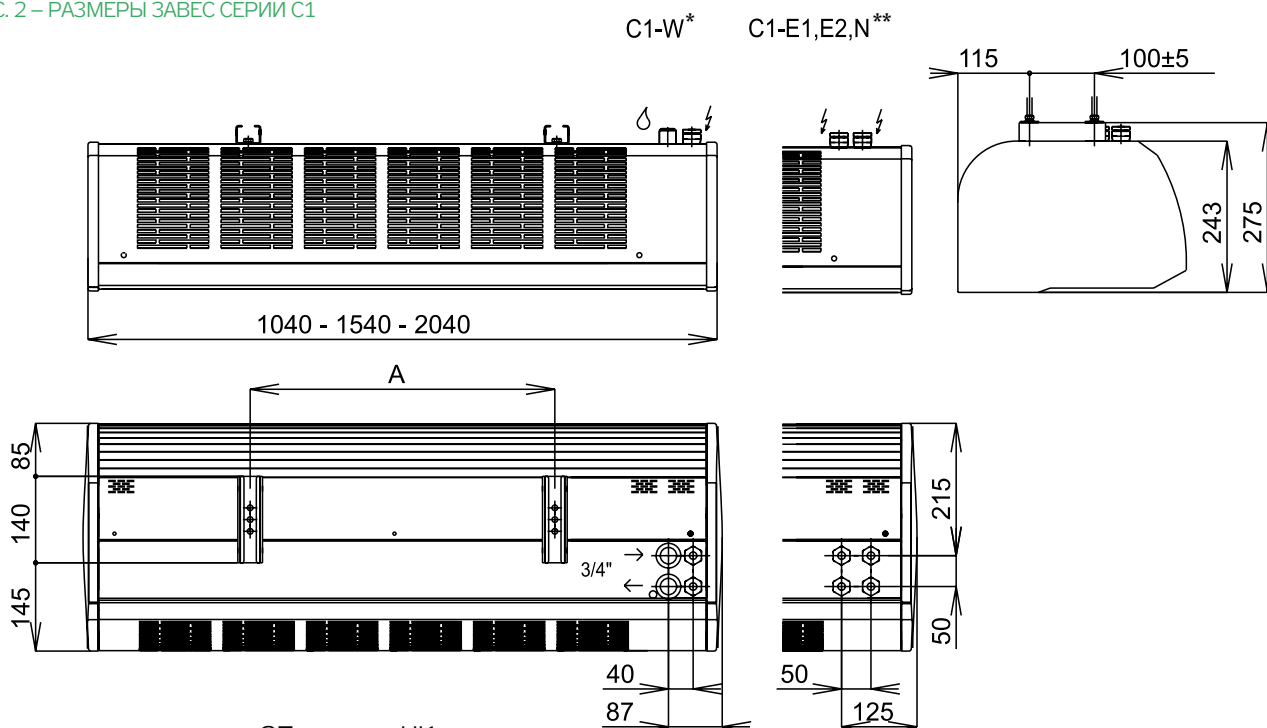
РИС. 2 – РАЗМЕРЫ ЗАВЕС СЕРИИ C1
