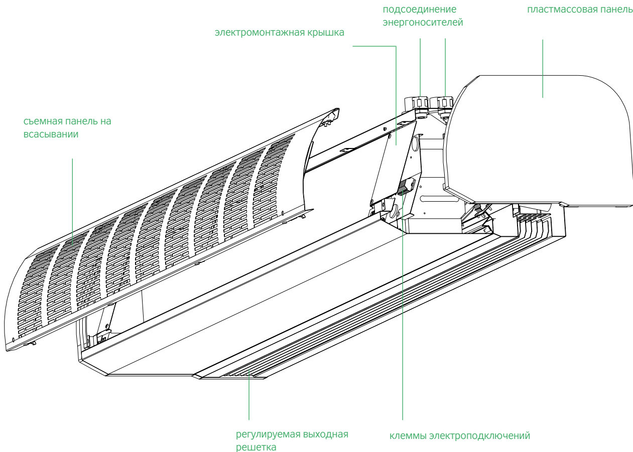
РИС. 2 – ОСНОВНОЕ ОПИСАНИЕ ЗАВЕС СЕРИИ C1
