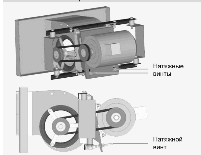
Рис. 15 – натяжка ремня
