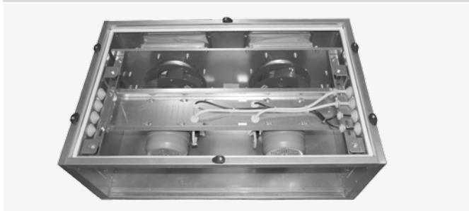
Рис. 13 – электропривод с двумя моторами
