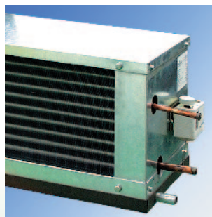
hűtő - beépített fagyvédelemmel és cseppvíztálcával
