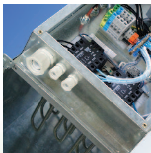
elektromos fűtő - beépített (SSR) kapcsolóelemmel
