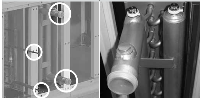
Рис. 17 – подключение энергоносителей
