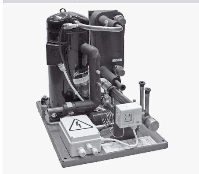
Рисунок 1 – Секция с встроенным блоком интегрированного охлаждения
