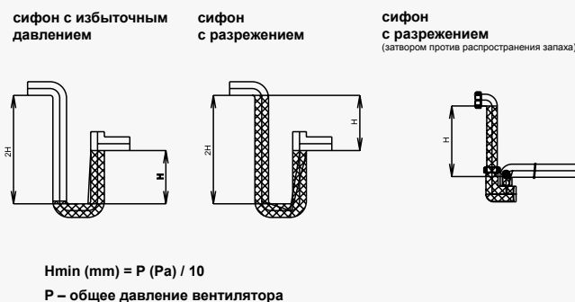
Рис. 21 – отвод конденсата
