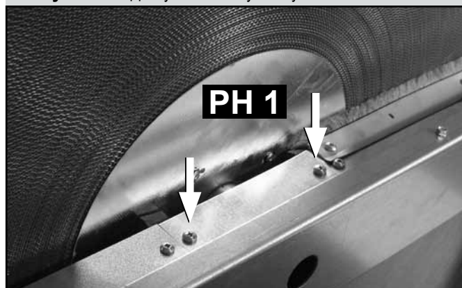
Рисунок 6 — Доступ к осевому болту колеса
