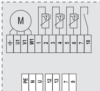
Рисунок 4 – Схема соединений регенератора
