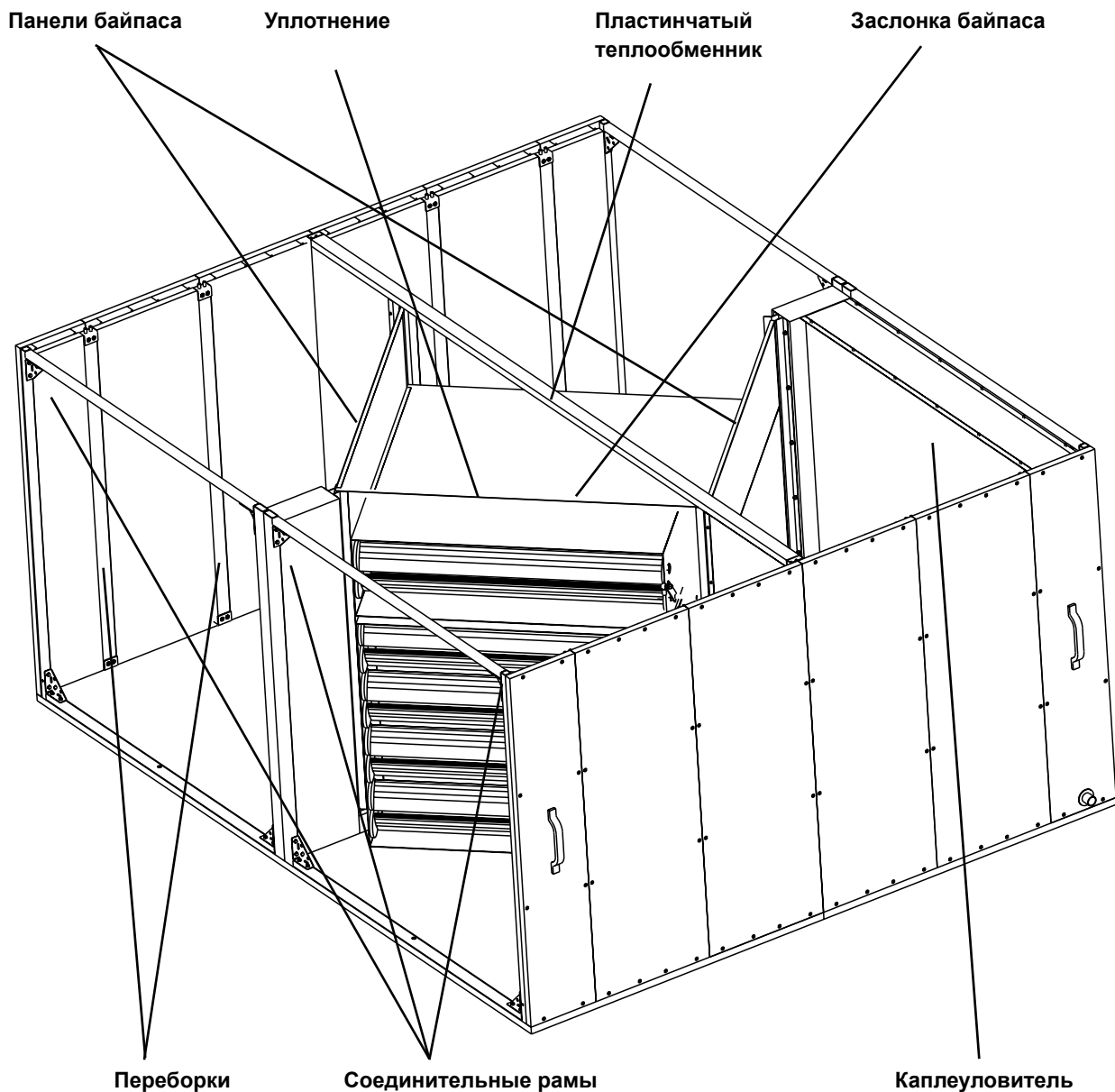
Рис. 2а – корпус секции XPXB 28/BS
