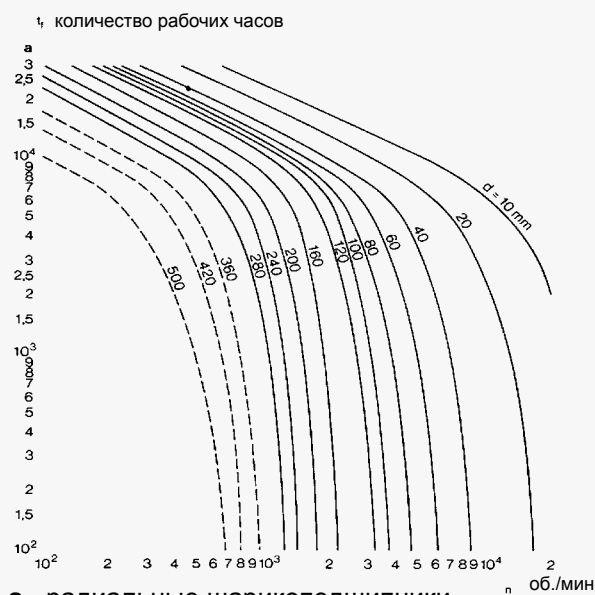
Рис. 24 — интервалы времени между смазкой
