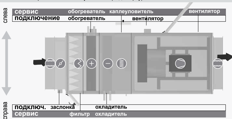
Рис. 1 – сторона исполнения установок (вид сверху)
