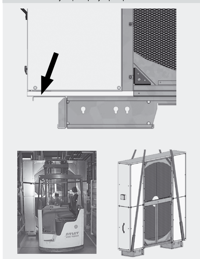
Рис 1 — Манипуляция с рекуператором
