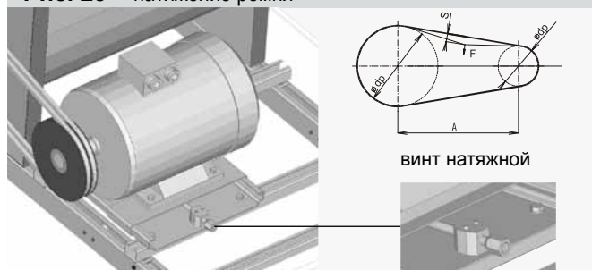
Рис. 23 — натяжение ремня
