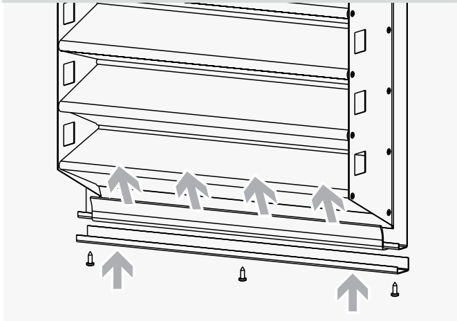
Рис.5 – окончание монтажа
