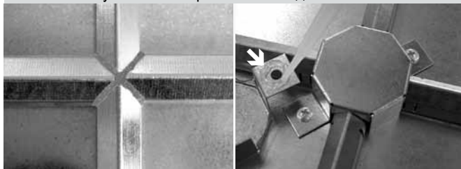
Рис. 13 – уплотнение крестового соединения
