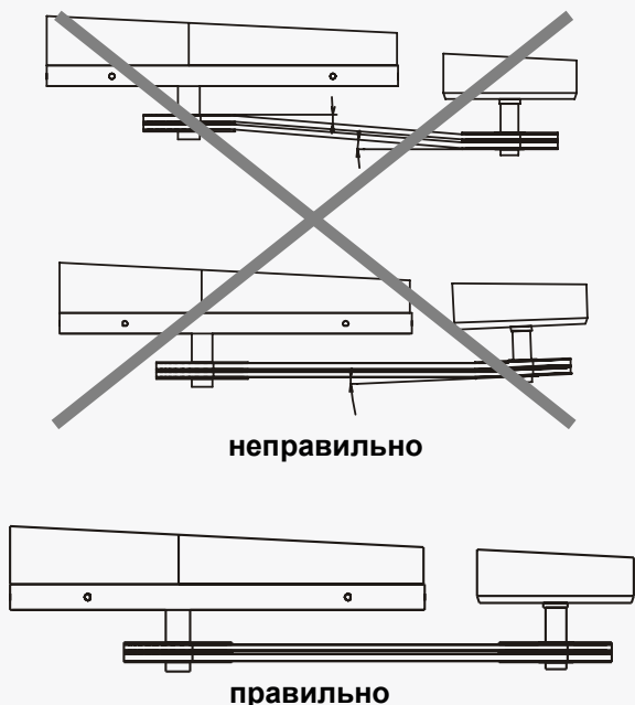
Рис. 25 – выравнивание шкивов
