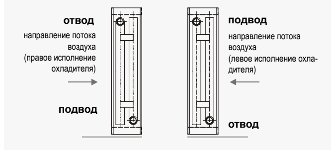
Рис. 18 – подсоединение теплообменников
