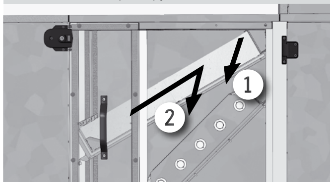
Рис. 2 – замена фильтрующих вставок
