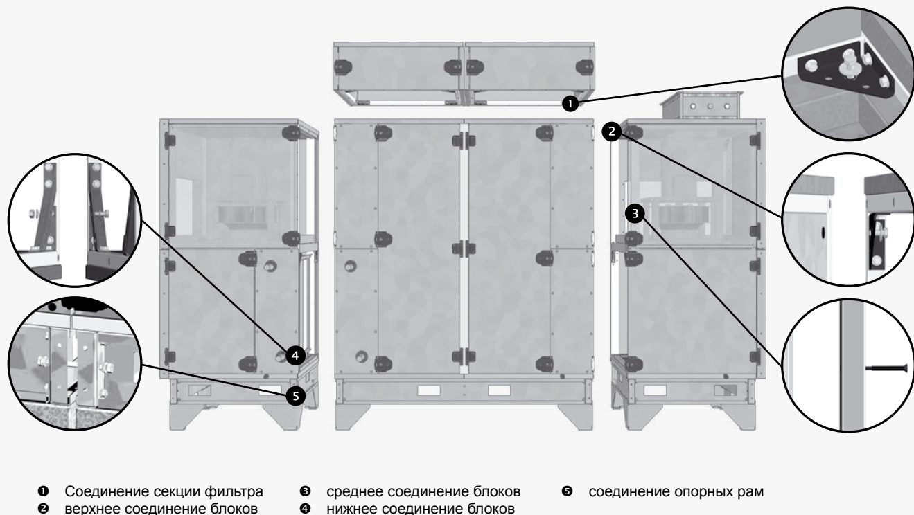
Рис. 1 – деталь внутреннего соединения блоков
