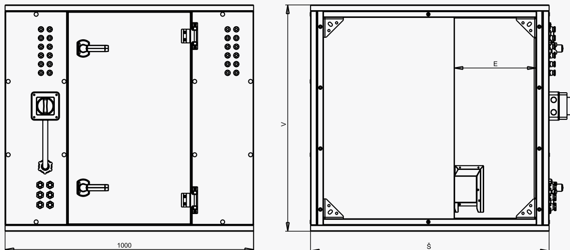
Рис. 3 — основные размеры секции
