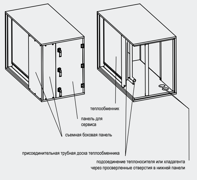
Рис. 19 – теплообменники в секции с закрытыми вводами
