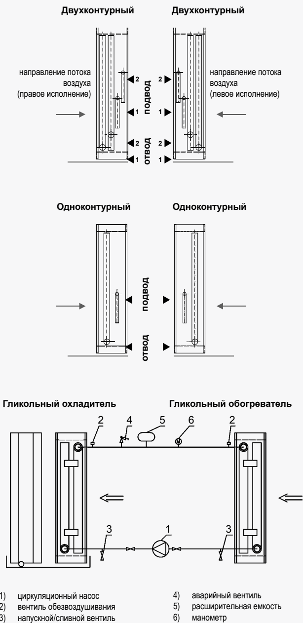
Рис. 20 – подсоединение испарителей
