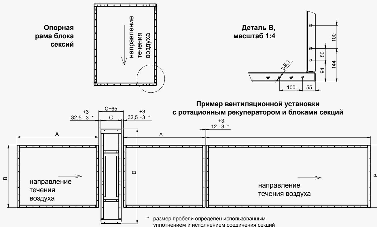
Рис. 6 – расположение опорной рамы
