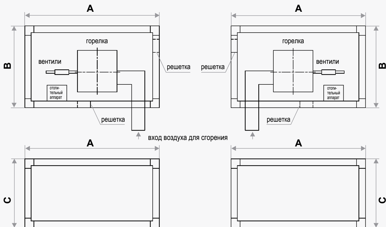
Рис. 1 – Размеры корпусов горелки с подогревом
