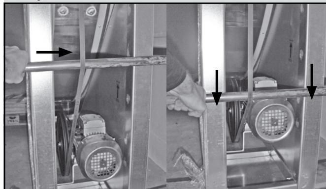
Рисунок 12 – Натяжка ремня
